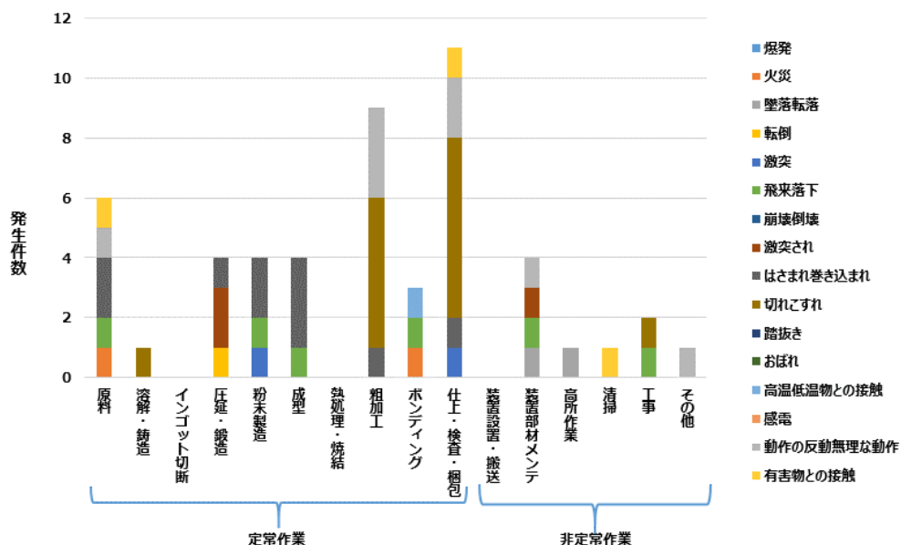
[図 II-8-10 ターゲット製造工程 工程別事故型発生件数(2005年～2021年)]
