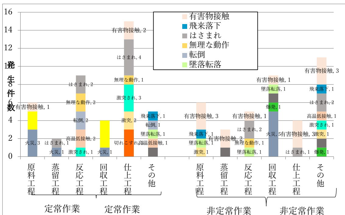
[図 II-2-5 多結晶シリコン製造工程別事故型発生件数 (2005 年～2021 年)]
