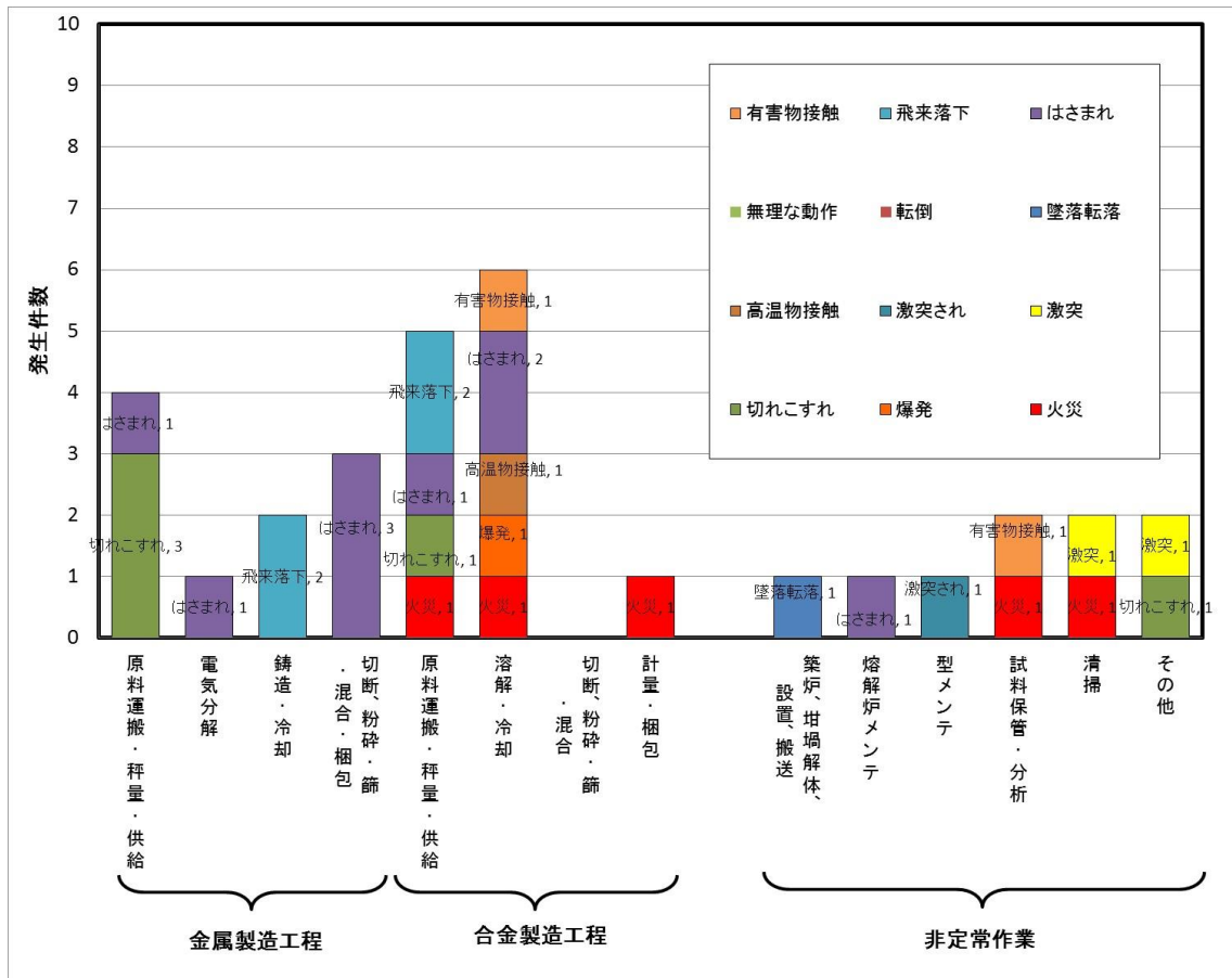
[図 II-4-11 金属・合金製造工程別事故型発生件数(2005年～2021年)]
