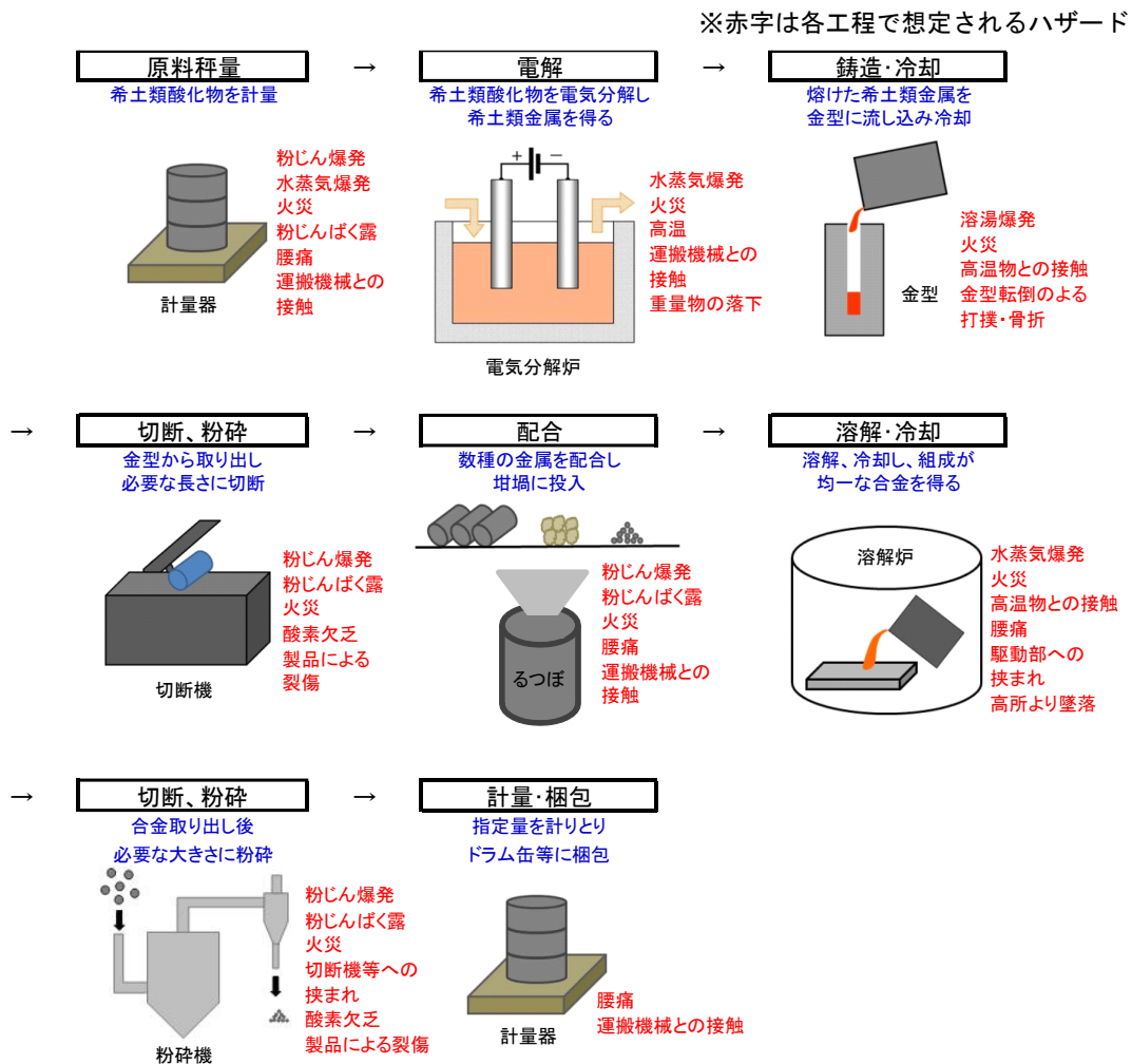
[図Ⅱ-4-13 金属・合金製造フロー]
