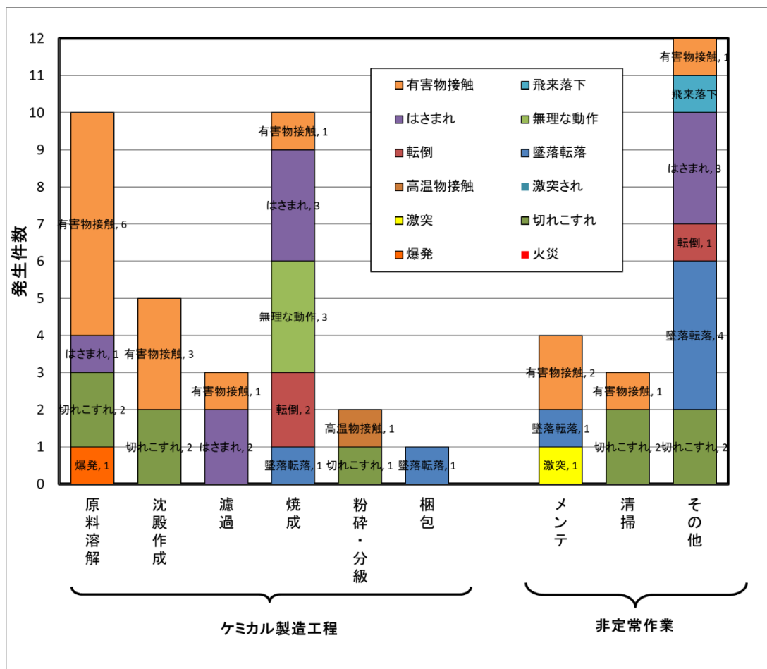
[図Ⅱ-4-10 ケミカル製造工程別事故型発生件数(2005年～2021年)]
