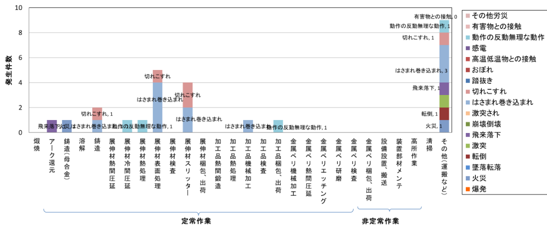
[図 II-12-10 ベリリウム製造工程 工程別事故型発生件数 (2005 年～2021 年)]
