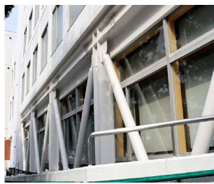
耐震化工事
