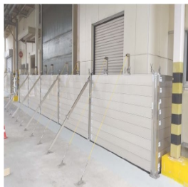
止水板
