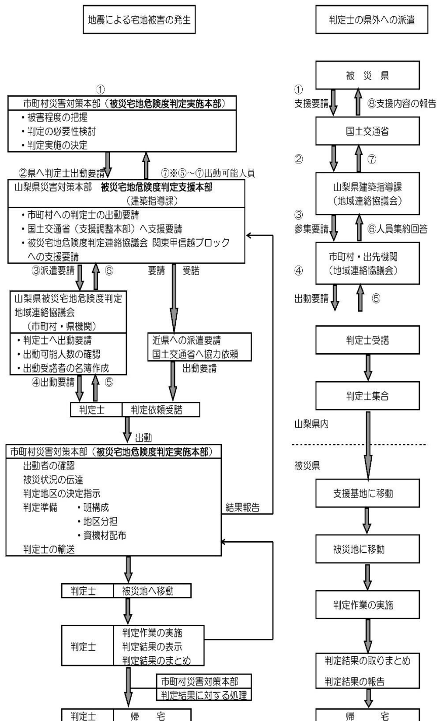
被災宅地危険度判定フロー
