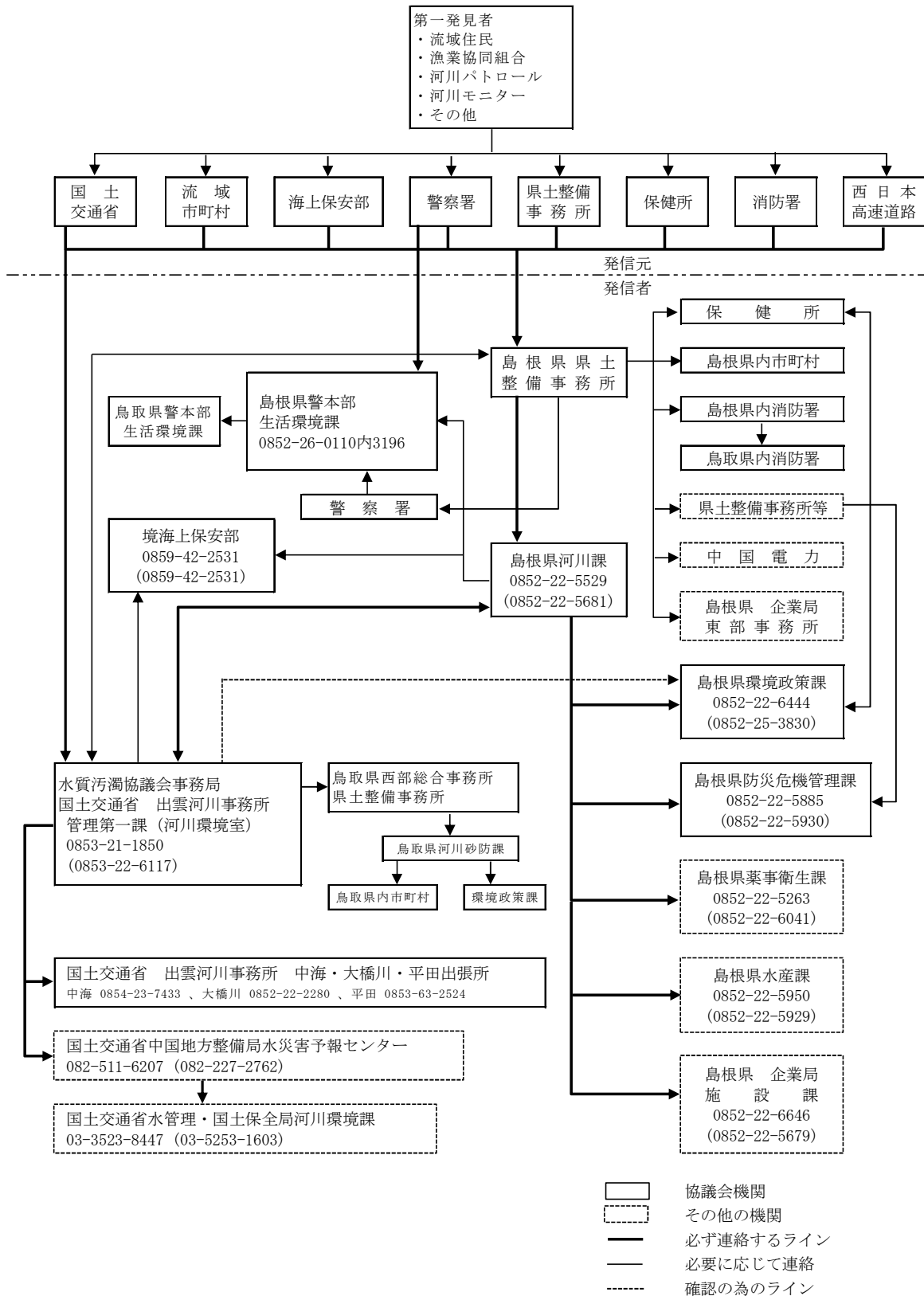
ア 河川、湖沼における流出油事故情報の収集伝達系統図 (斐伊川水系水質汚濁防止連絡協議会)
