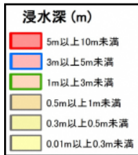
図7 津波浸水予測図
