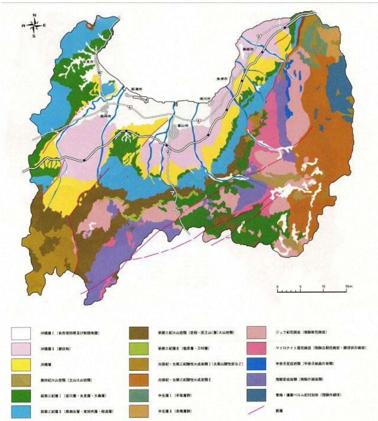
図2 富山県地質図
