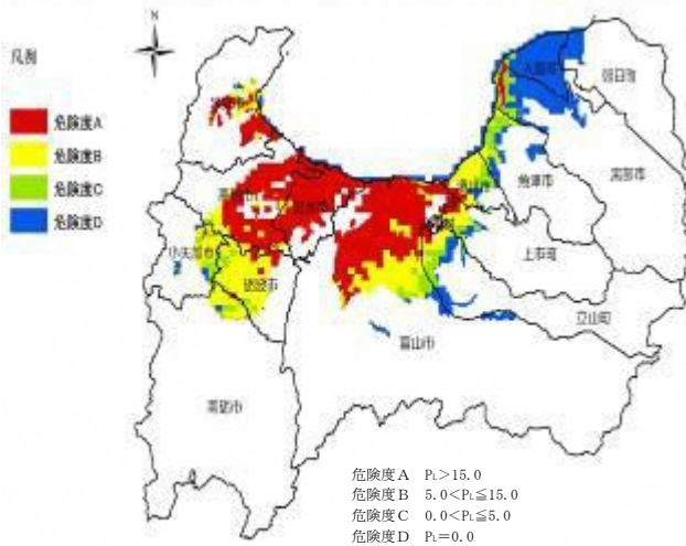
图 5.2 呉羽山断層地震液状化判定結果図
