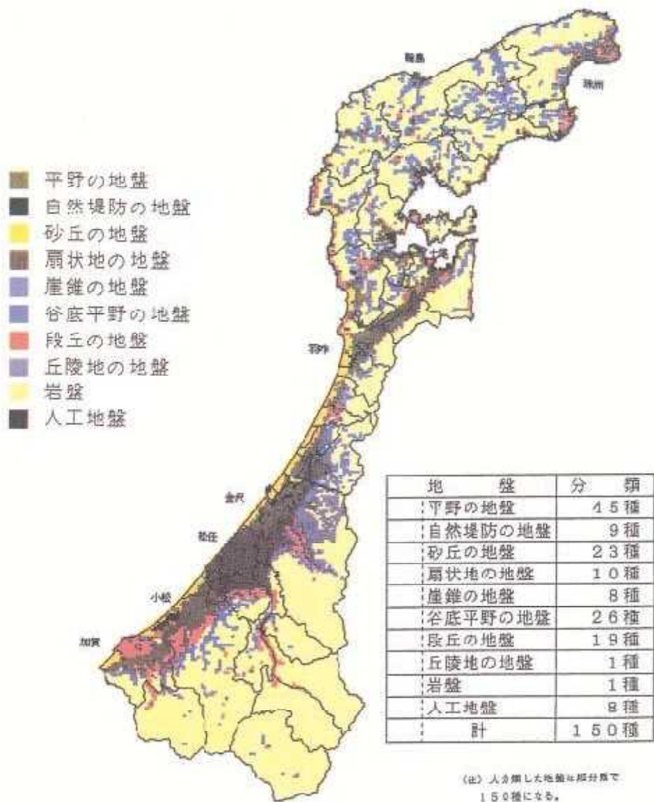
図 地盤種の大分類と分布
