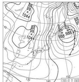
図1 山雪型の概念図（左）と気圧配置（右）（参考〔2〕）
