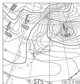
図2 里雪型の概念図（右）と気圧配置（左）（参考〔2〕）
