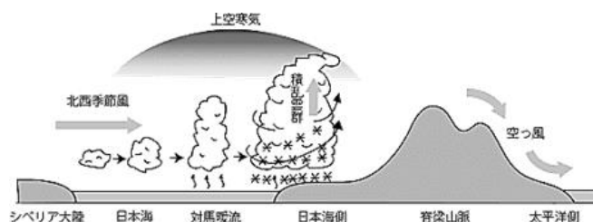
図2 里雪型の概念図（右）と気圧配置（左）（参考〔2〕）
