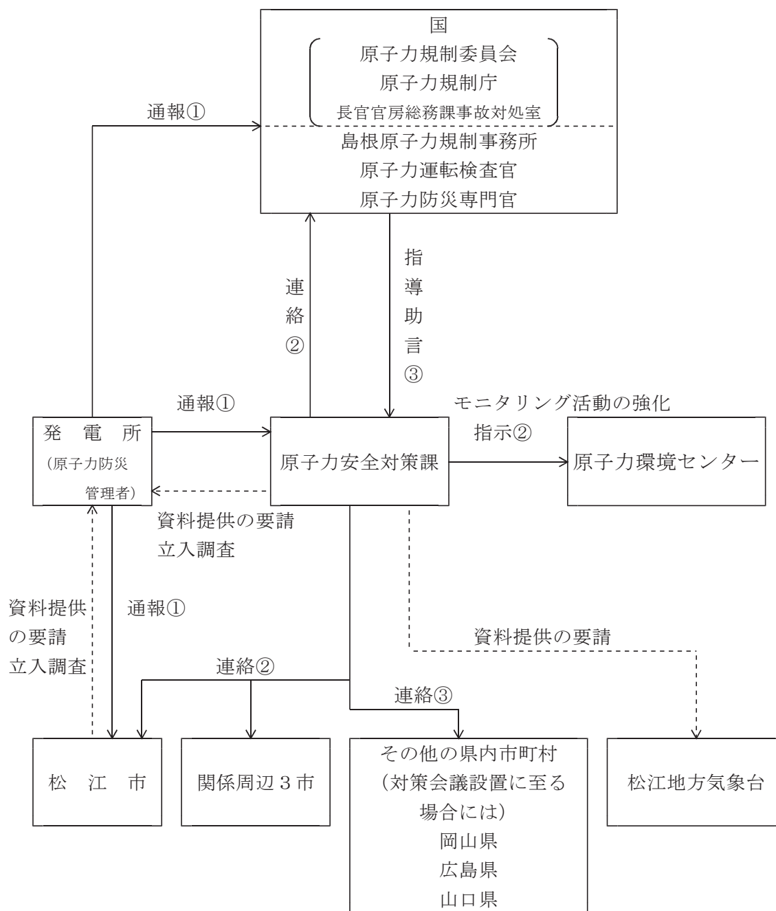
図2 発電所異常時連絡系統図
