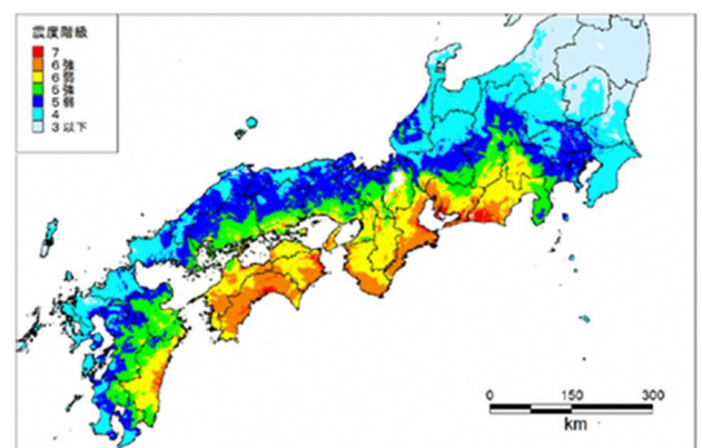
南海トラフの巨大地震による津波高・震度分布等 南海トラフ地震の想定震度分布（H24.8.29 南海トラフ巨大地震対策検討ワーキンググループ）
