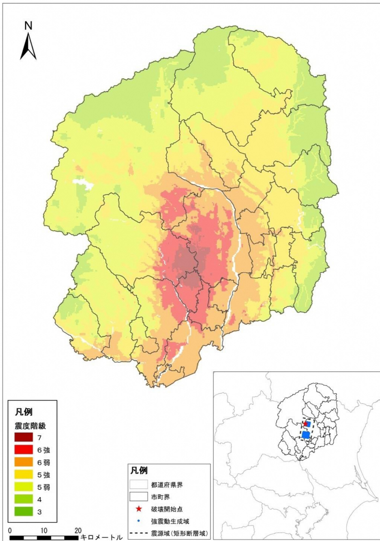
○県庁直下地震M7.3の震度分布図
