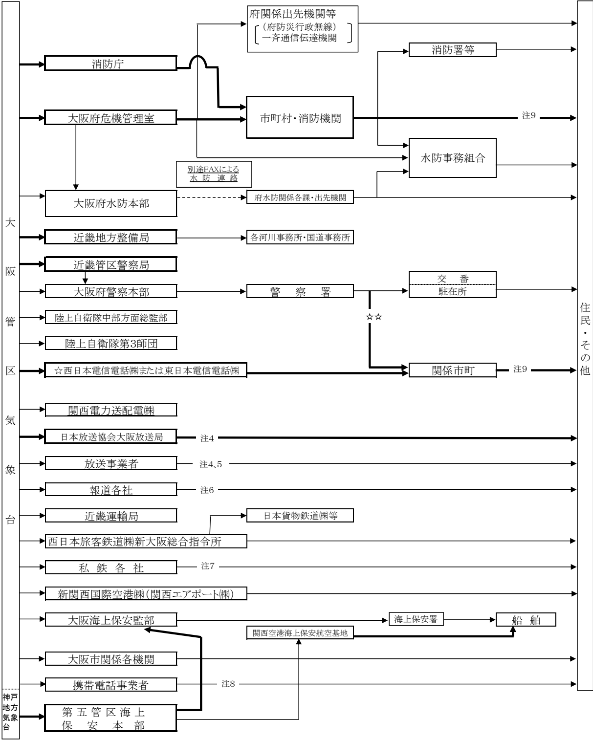
[別図1-1] 津波予警報等の関係機関への伝達経路
