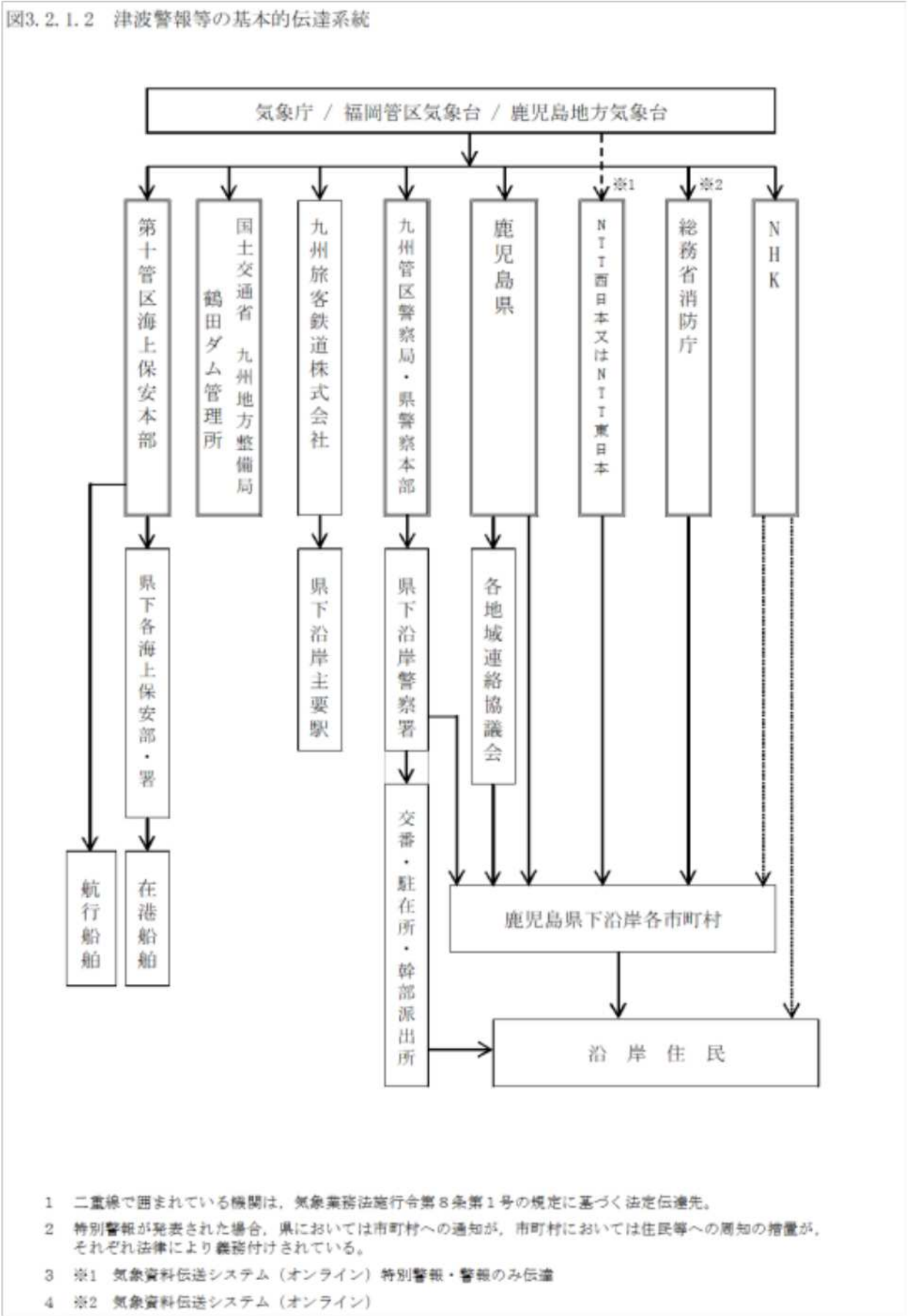
図3.2.1.2 津波警報等の基本的伝達系統
