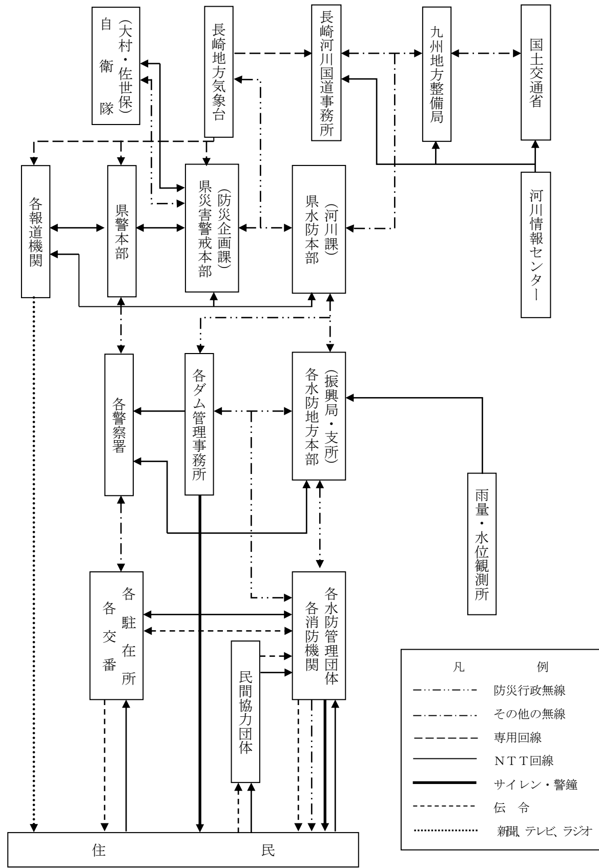
水防情報伝達系統図
