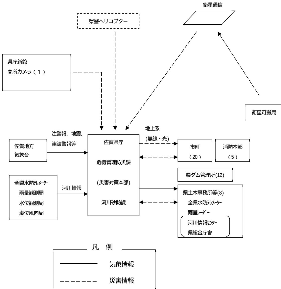
【 防 災 情 報 連 絡 系 統 図 】
