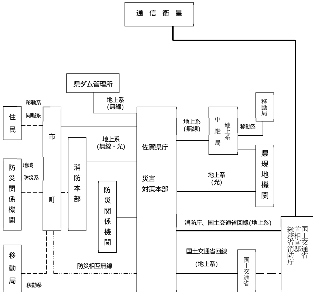
【通信系統図】
