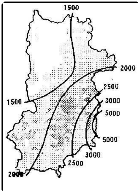
図3 県内の年平均降水量分布
