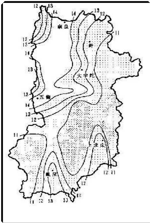
図2 県内の年平均気温分布
