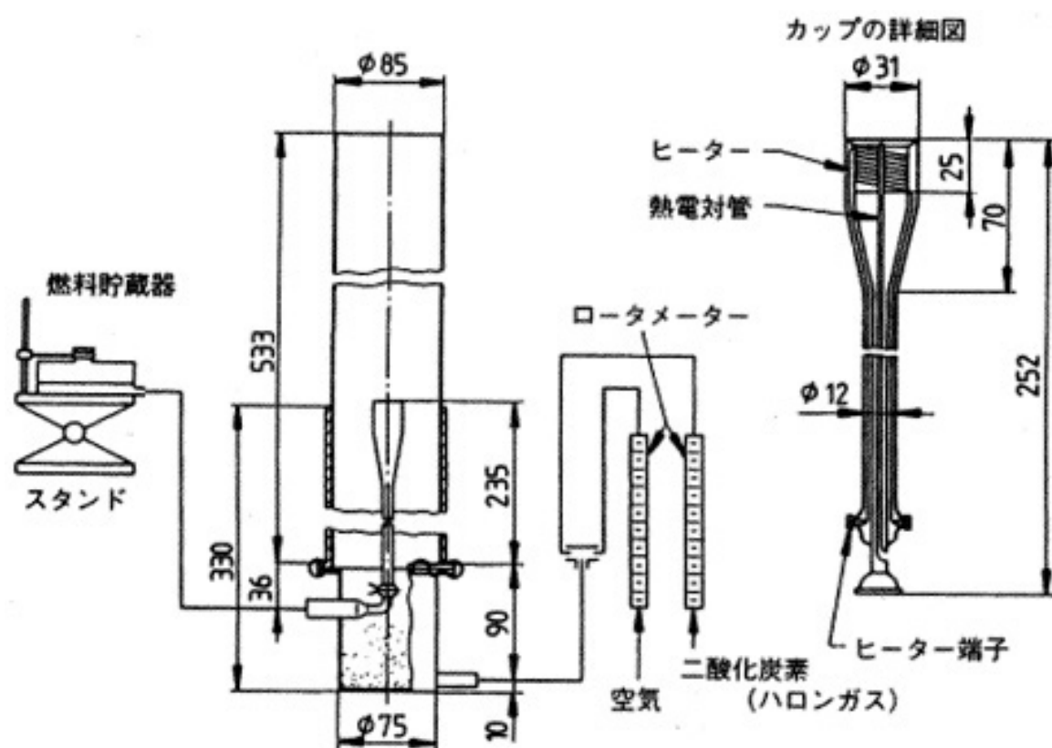
図1 カップ燃焼装置
