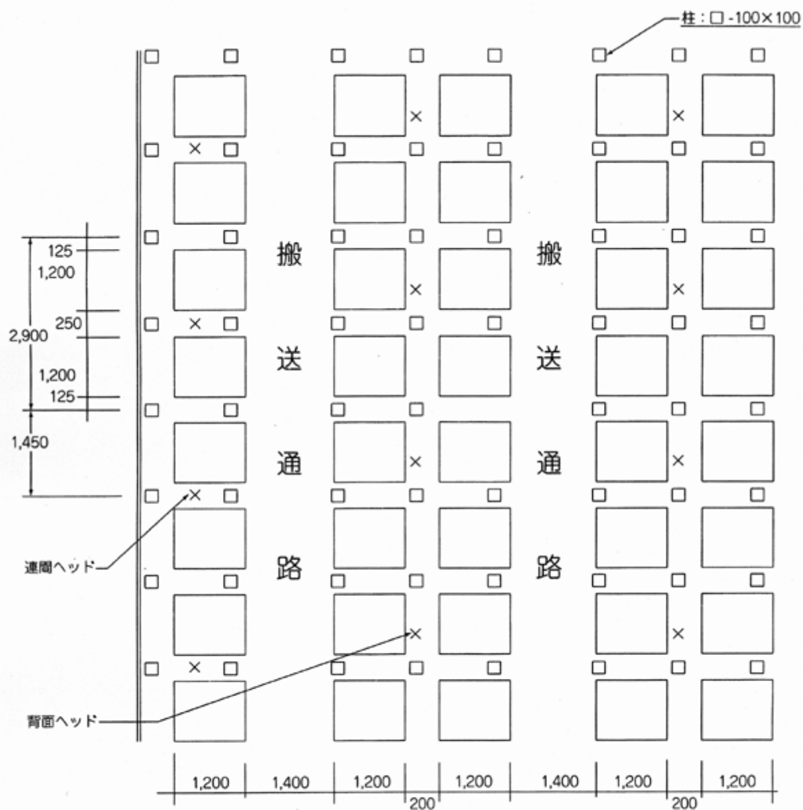
平面 (レベル1、3、5配置)
