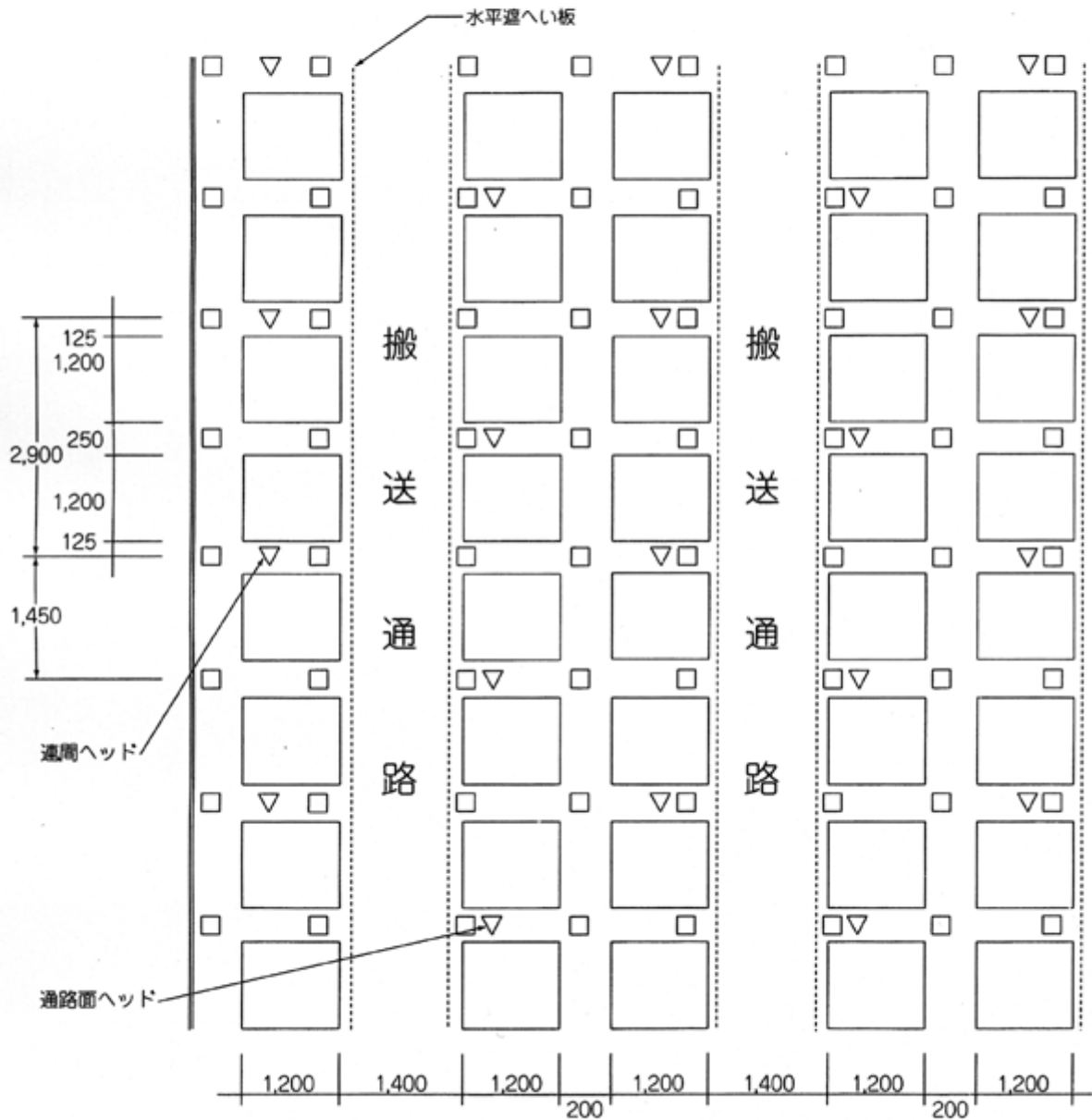
平面 (レベル2、4、6配置)
