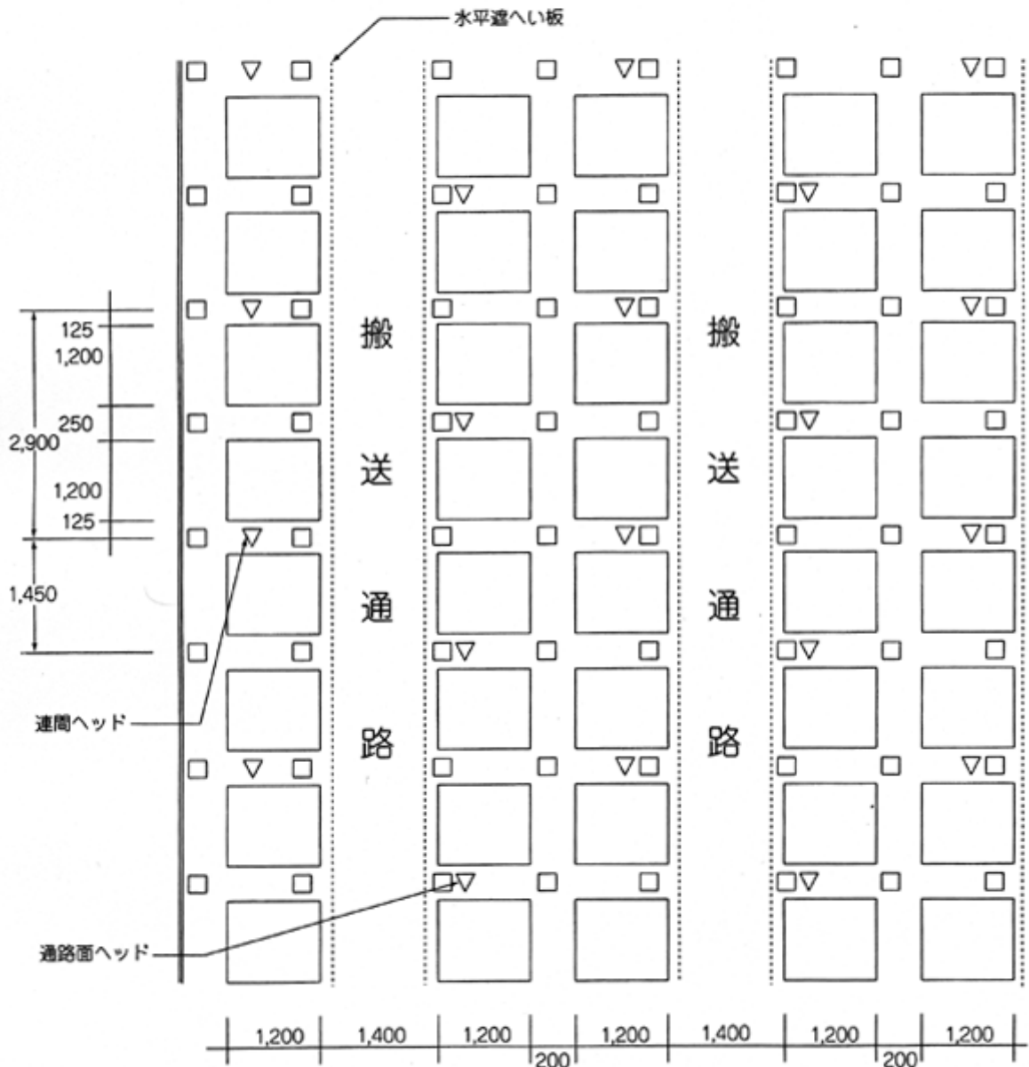
平面 (水平遮へい板直下-レベル2、4、6配置)
