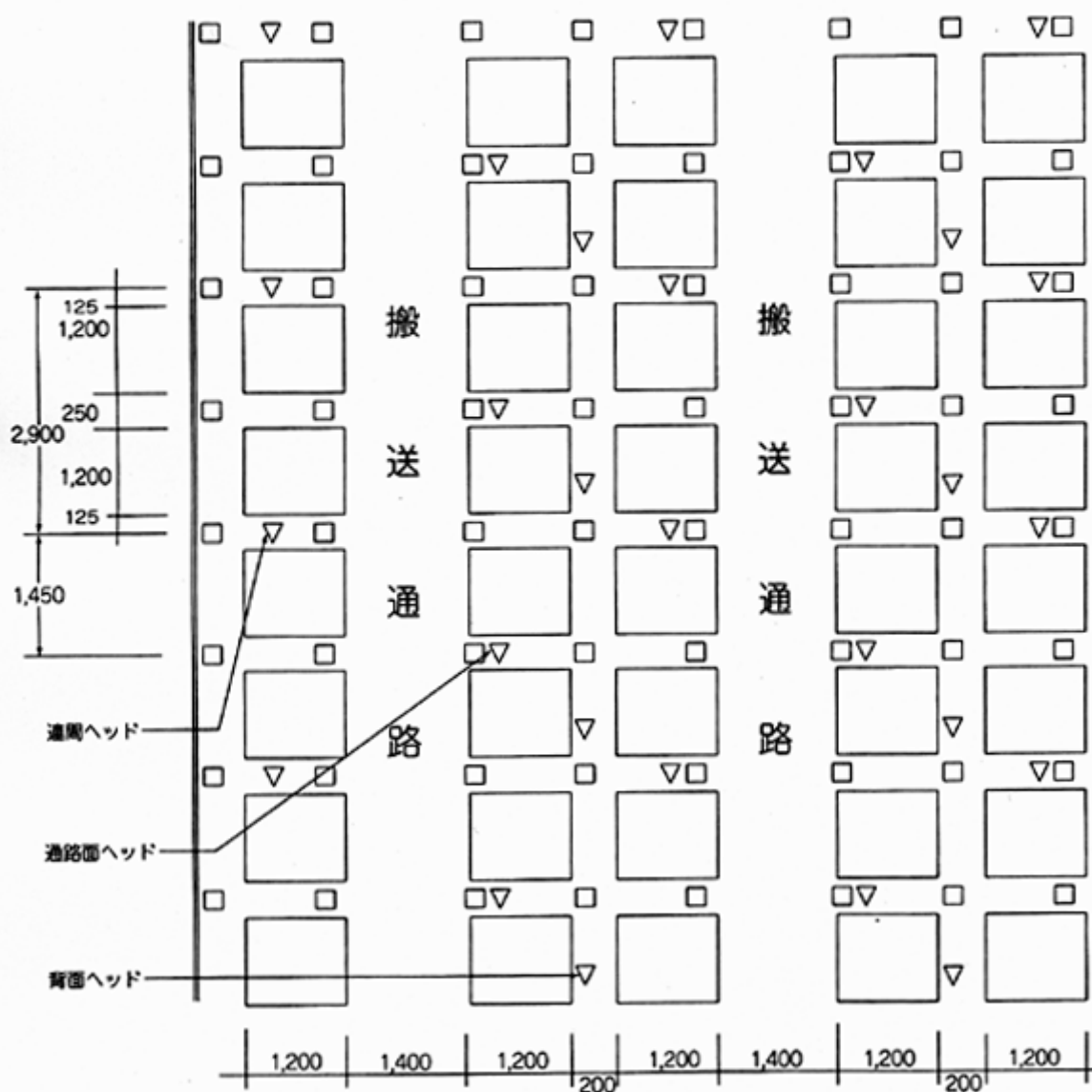
平面 (レベル2、4、6配置)
