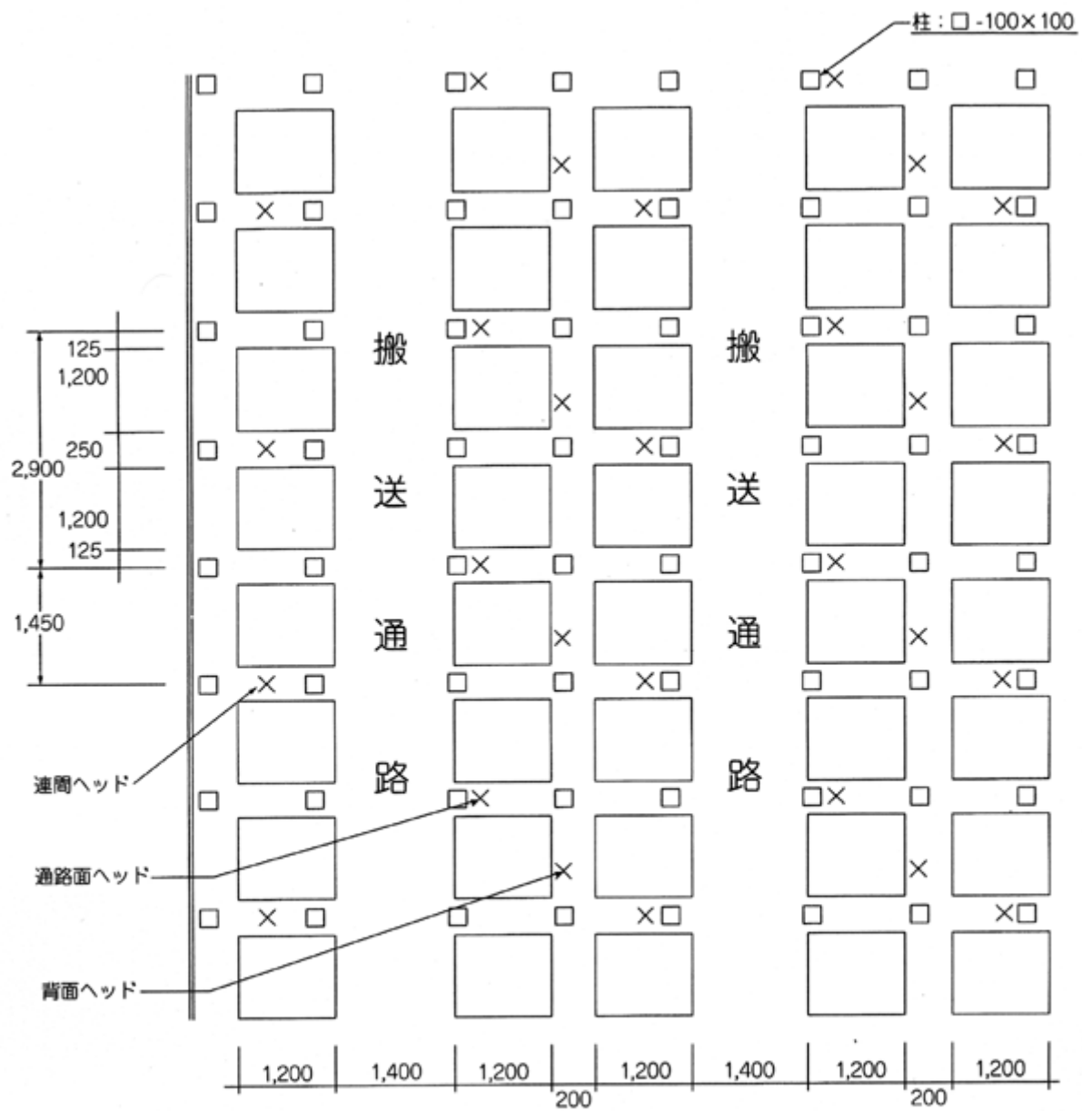
平面 (レベル1、3、5配置)
