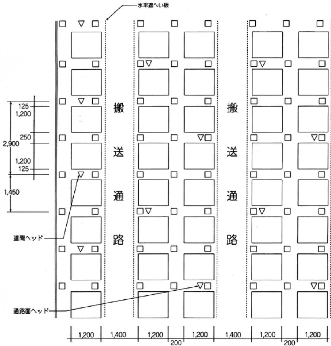
平面 (水平遮へい板直下-レベル2、4配置)
