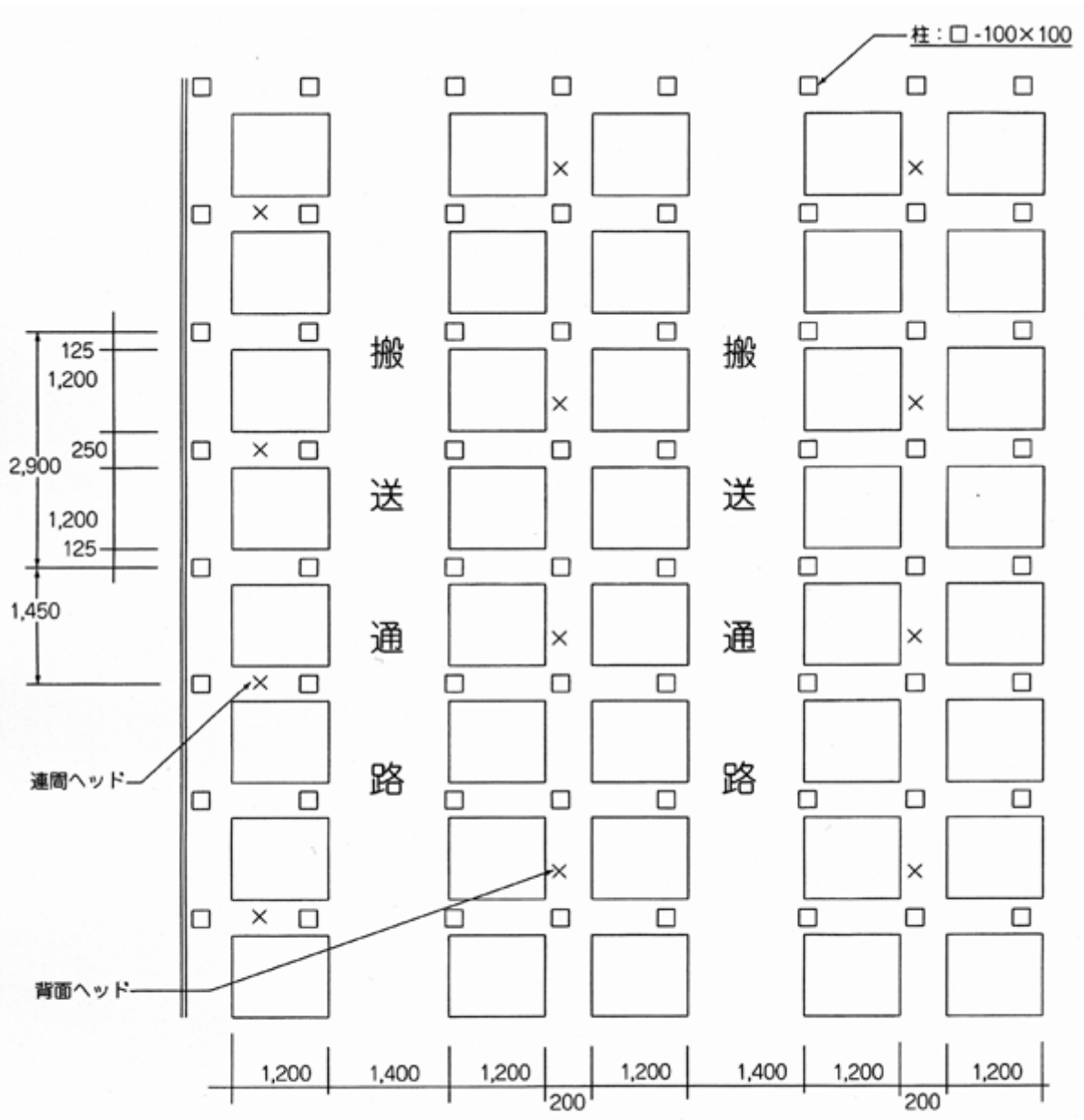
平面 (レベル1、3配置)
