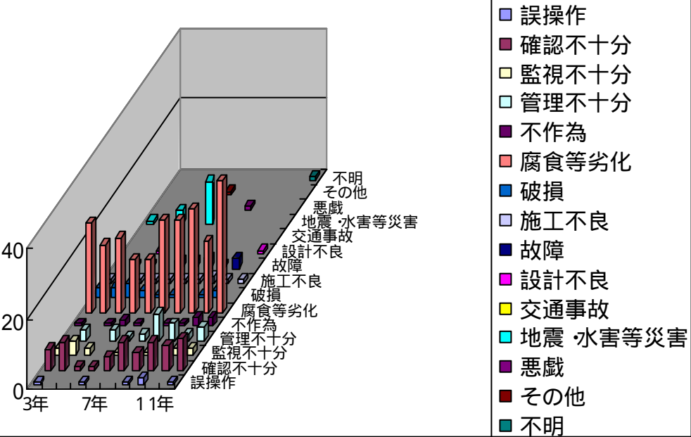
地下タンクにおける漏えい発生要因
