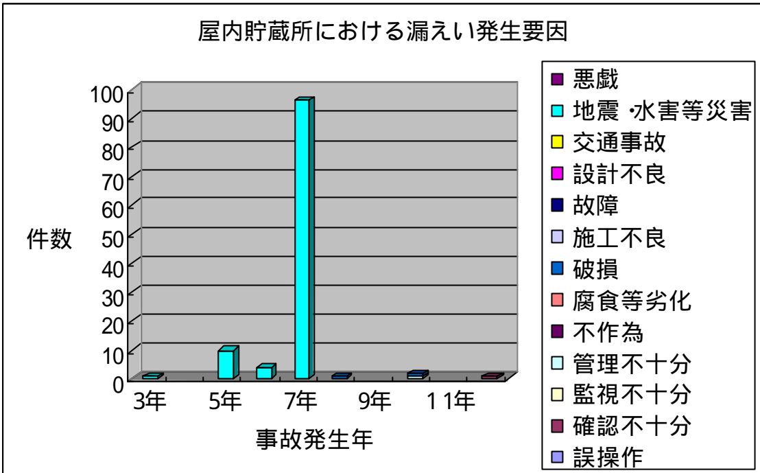
屋内貯蔵所における漏えい発生要因
