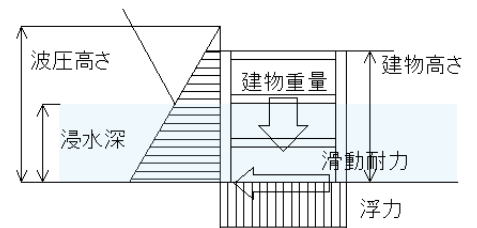
(B) 波圧高さが建物高さを上回る 波圧分布(台形)
