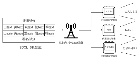
図 3 多言語対応のイメージ (右写真は屋内受信機 (試作機) の言語設定画面)
