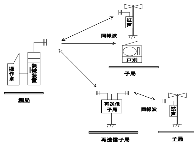
図 13 親局＋再送信子局＋子局構成
