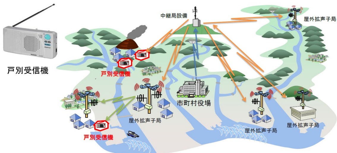
図5 戸別受信機を用いた防災行政無線等の構成イメージ
