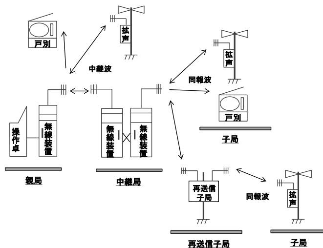
図 14 親局＋中継局＋再送信子局＋子局構成
