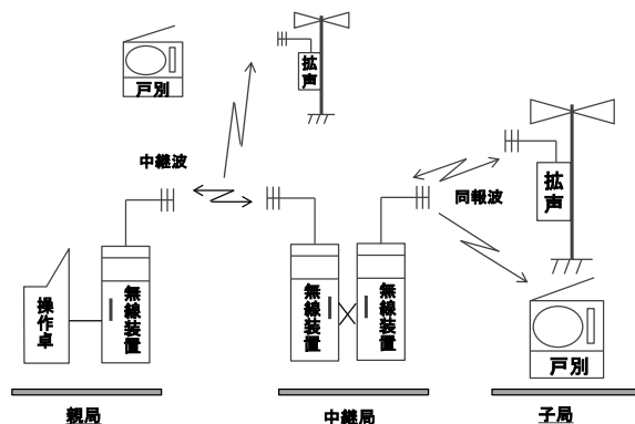
図 12 親局＋中継局＋子局構成
