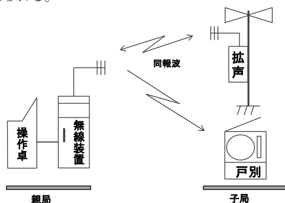
図 11 親局＋子局構成
