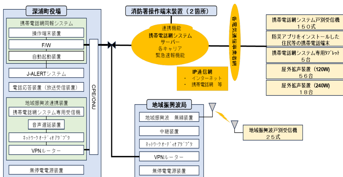
<図1・深浦町防災行政情報伝達システムの概要>
