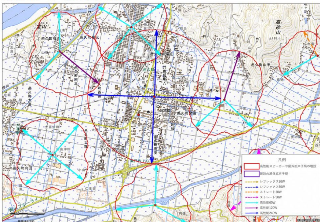
<図6・新旧スピーカー音達範囲（右図中心の円が高性能スピーカー音達範囲）>
