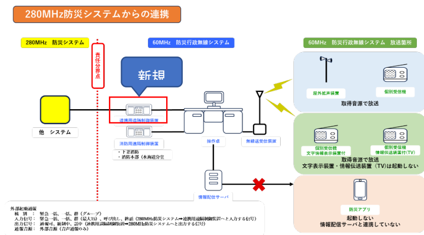
＜図４・システム連携と責任分界点＞ （出典 常総市提供資料をもとにイメージ図作成）
