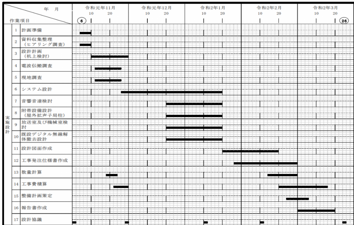
<図3・システム設計スケジュール>
