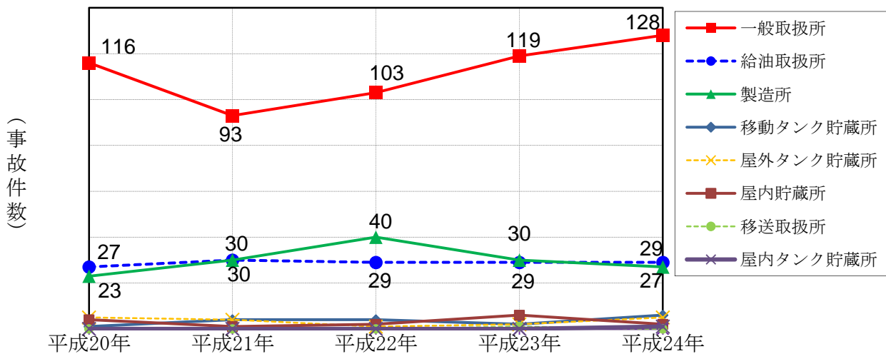
第3図 危険物施設における火災事故件数の推移（最近の5年間）
