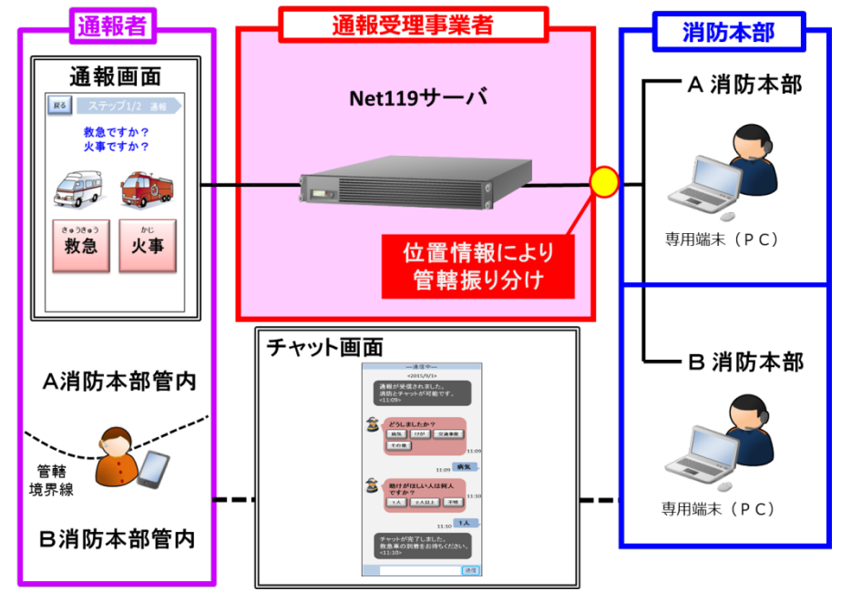
Net119システム概要図
