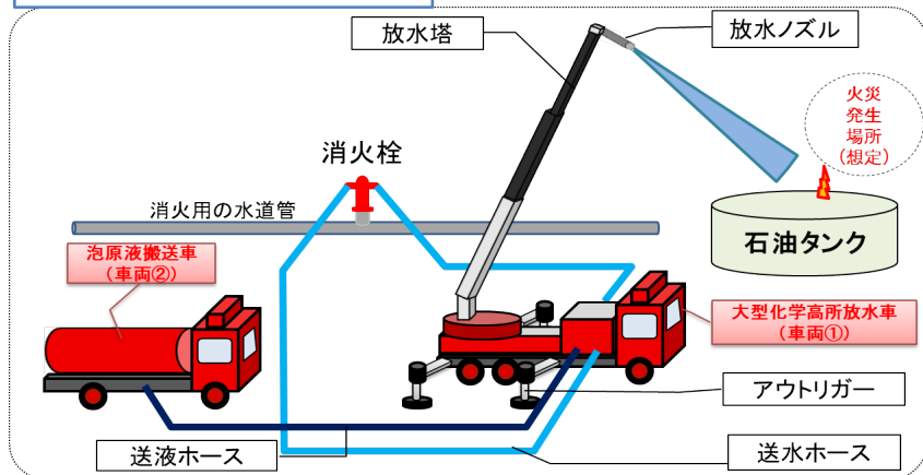
大型化学高所放水車 + 泡原液搬送車
