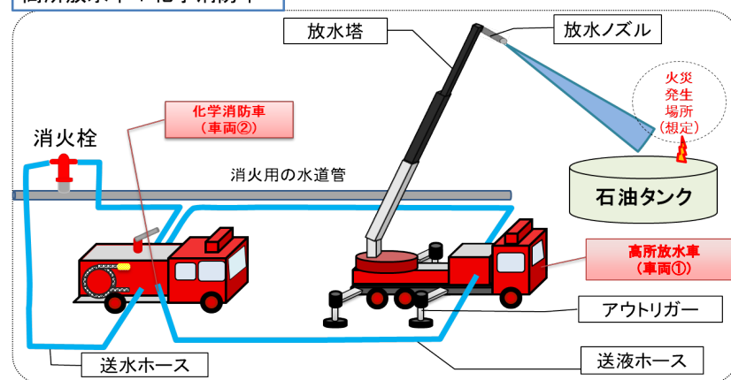
高所放水車 + 化学消防車
