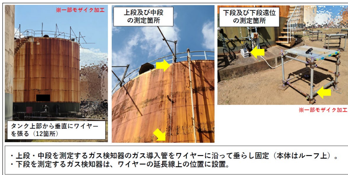
図2-10 ガス検知器設置状況（浮き蓋付きの屋外貯蔵タンク）
