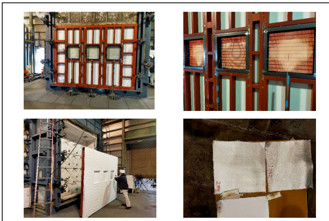
図4－12 耐火性能試験の状況
