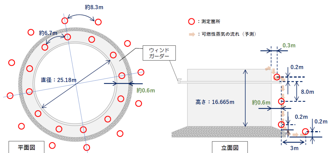
図2-7 測定箇所詳細（浮き屋根を有する屋外貯蔵タンク）
