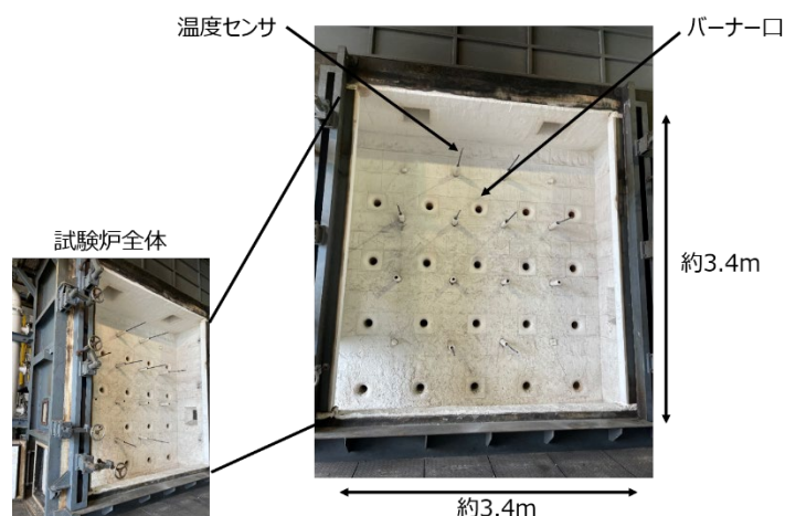
図 4－9 燃焼試験炉
