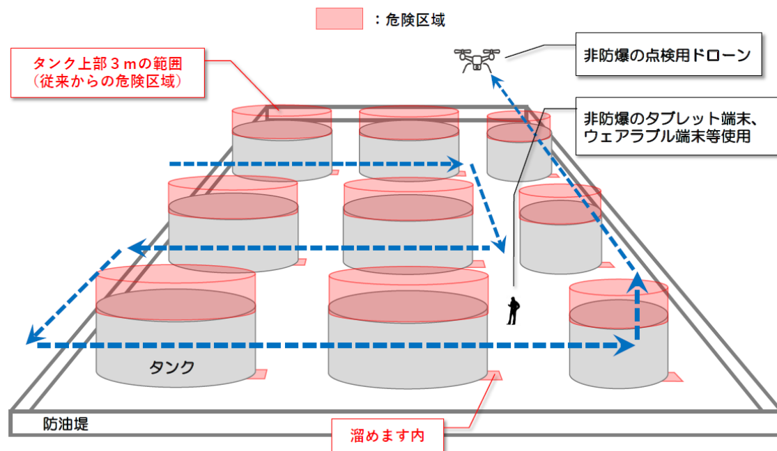
図2-14 定常時における非防爆機器の活用イメージ
