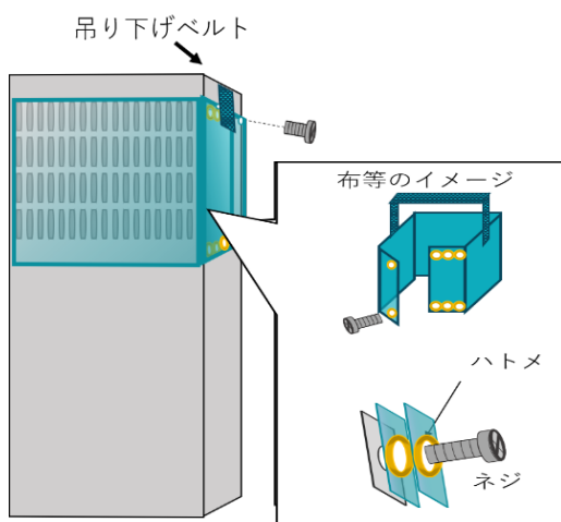
図4-17 〔キュービクルに布をかける方法（耐火性を有するベルトで吊り下げベルト等で固定する方法）〕
