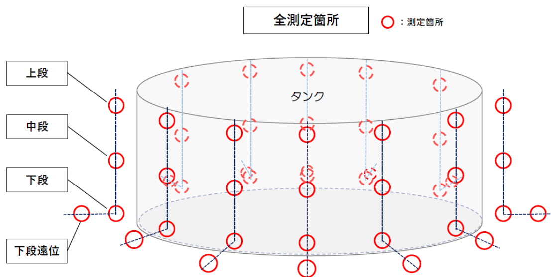
図 2 - 6 測定箇所
