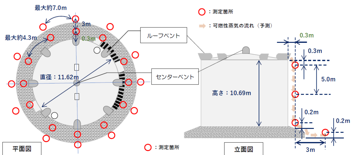
図2-9 測定箇所詳細（浮き蓋付きの屋外貯蔵タンク）
