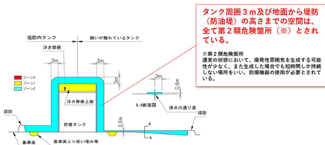
図 2-15 ユーザーのための工場防爆ガイド（浮屋根式可燃性液体備蓄タンクの例）
