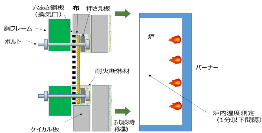
図 4 - 11 燃焼試験のイメージ
