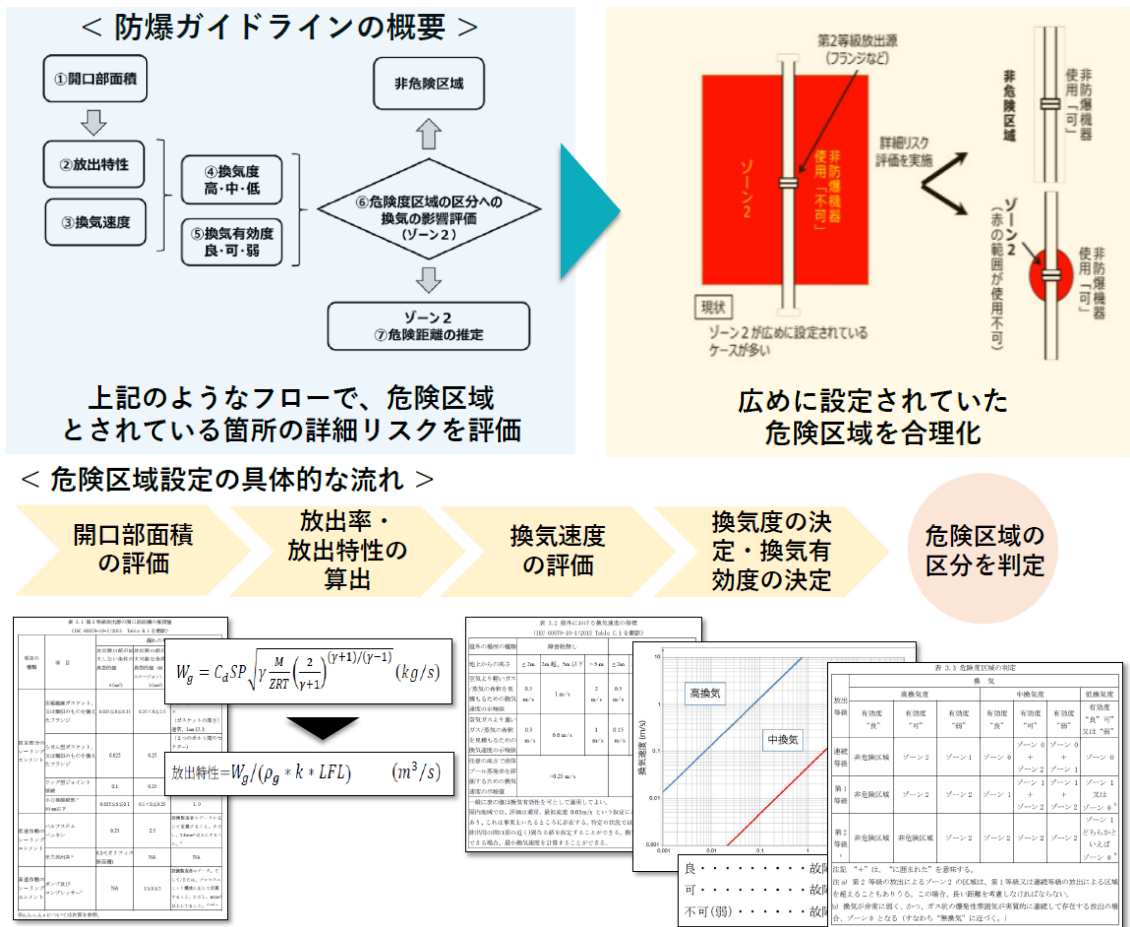
図 2-1 防爆ガイドラインの概要と危険区域設定の具体的な流れのイメージ
