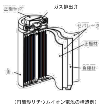
図4-2 リチウムイオン蓄電池の構造例
