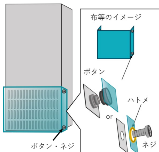
図4-15 〔換気口部分を覆う方法〕
