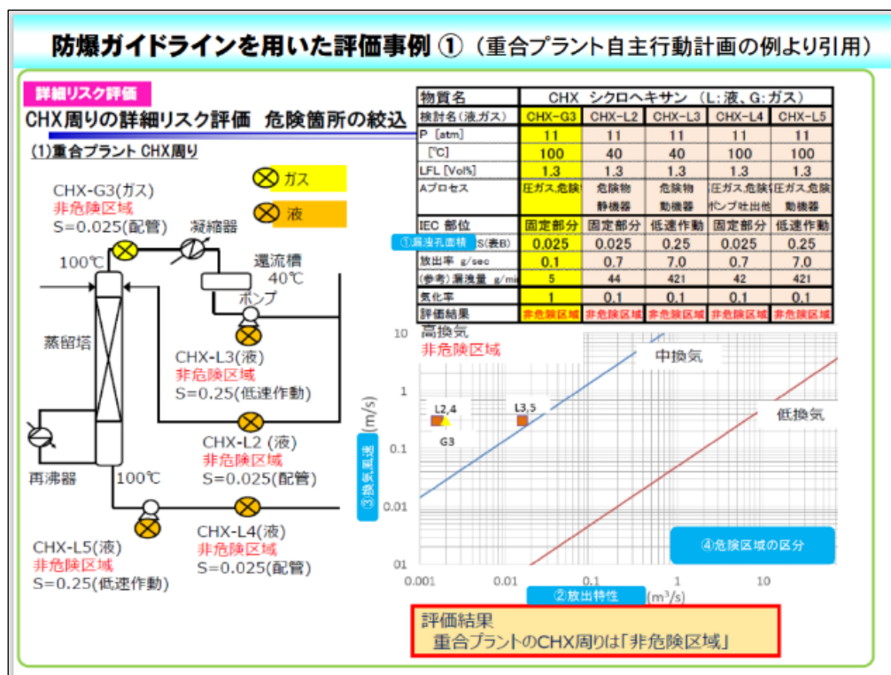
図 2 - 2 重合プラント周りの評価事例
