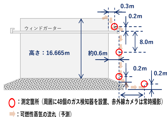
フローティングルーフタンク (ガソリン)
