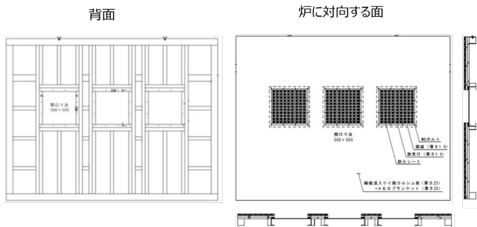
図 4 - 10 試験体について
