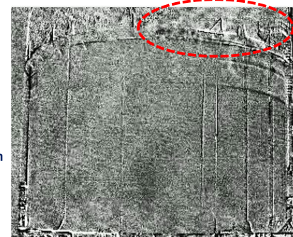
赤外線カメラでの撮影結果
