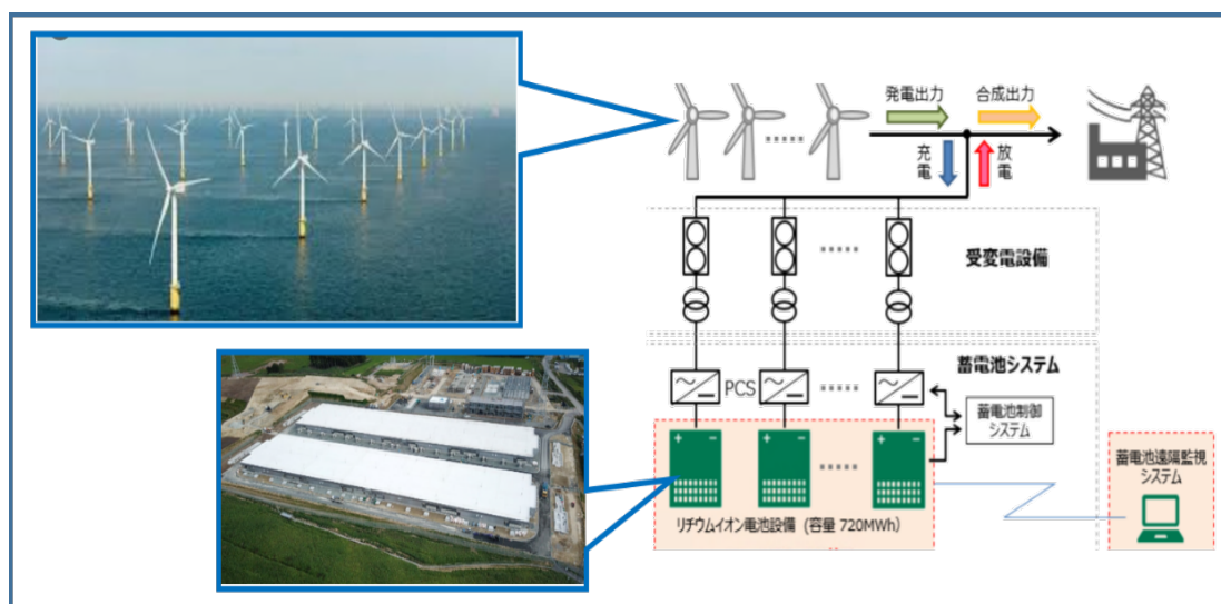
図4-1 リチウムイオン蓄電池の活用イメージ
