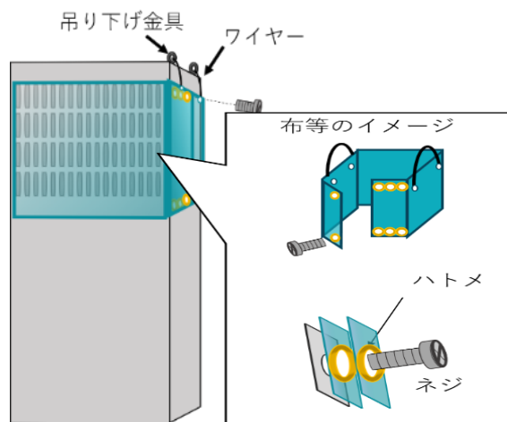
図4-16 〔キュービクルに布をかける方法 (耐火性を有するワイヤーで吊り下げベルト等で固定する方法)〕
