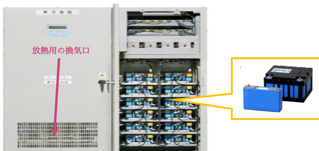
図 4－5 キュービクル式リチウムイオン蓄電池
