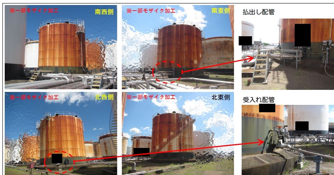
図 2 - 5 浮き蓋付きの屋外貯蔵タンク外観
