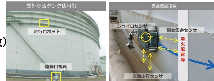
【点検ロボットを用いたタンク点検のイメージ図】
