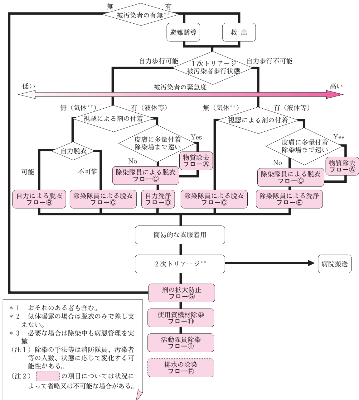
化学テロ災害除染活動フローチャート（例）
