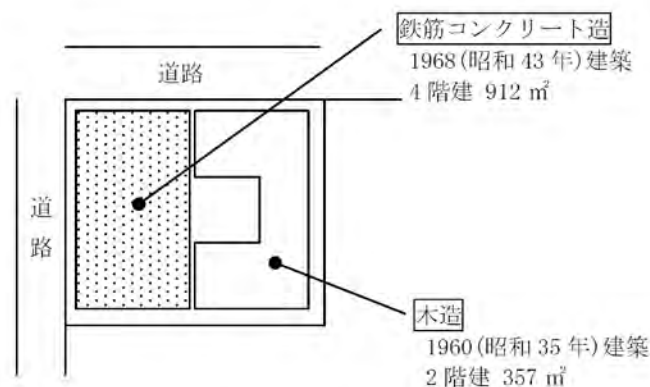
図1 建物配置図（福山市建築物査察等適正化対策委員会最終取りまとめより）
