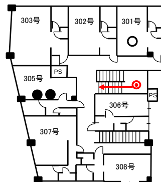
【3階平面図】
