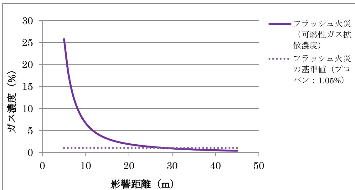
図2-3-1 プロパンの拡散火炎が伝ばし得る範囲の評価
