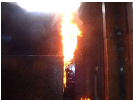
写真3-2-3 噴出火災
