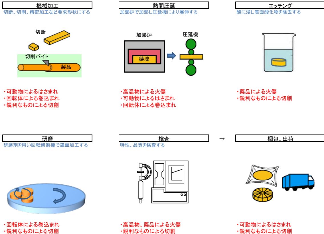
[図Ⅱ-12-13 ベリリウム製造フローと主な潜在危険性（金属ベリリウム加工品）]
