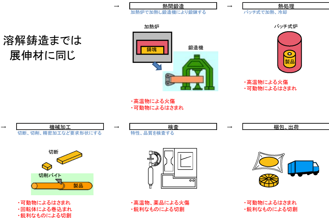
[図Ⅱ-12-12 ベリリウム製造フローと主な潜在危険性（ベリリウム銅加工品）]
