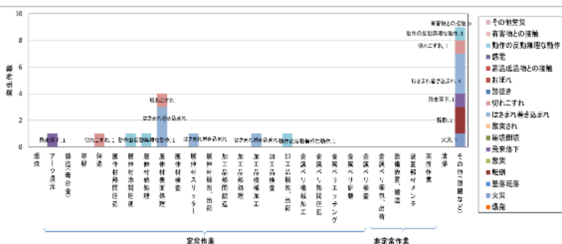
図Ⅱ-12-10 ペリリウム製造工程 工程別事故型発生件数 (2005年～2020年) ]
