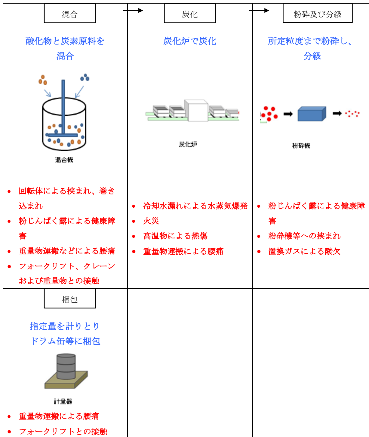
[図 II-6-2 タンタル炭化物製造フローとハザード]
