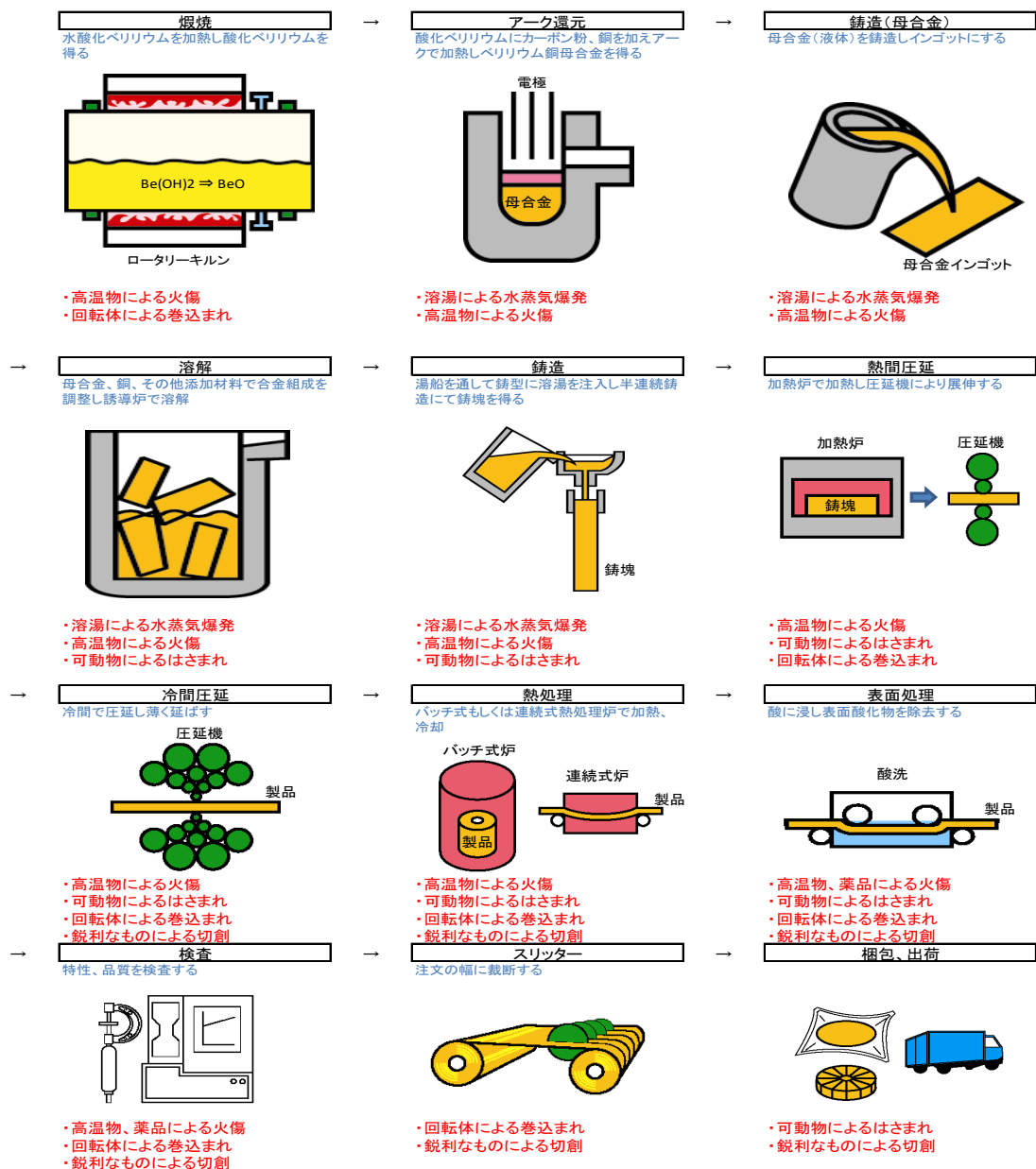
図Ⅱ-12-11 ベリリウム製造フローと主な潜在危険性(ベリリウム銅合金展伸材)
