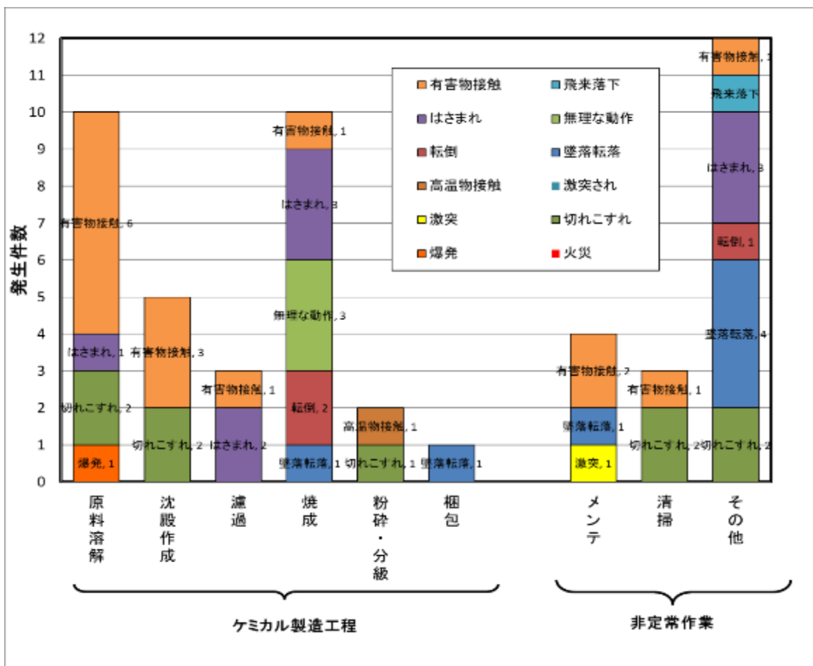
[図Ⅱ-4-10 ケミカル製造工程別事故型発生件数（2005年～2020年）]
