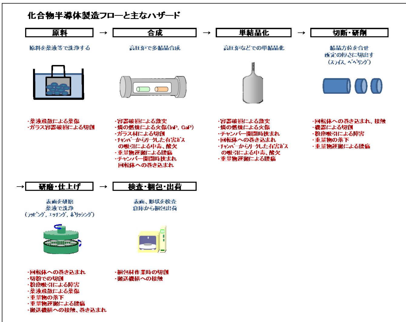
[図 II-10-6 化合物半導体製造フローと主な潜在危険性 (ハザード)]
