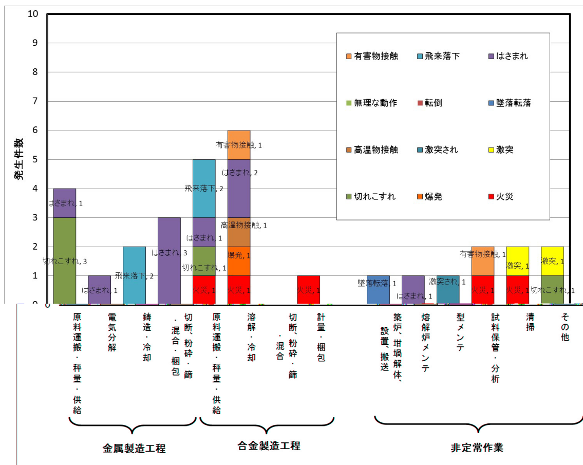
[図Ⅱ-4-11 金属・合金製造工程別事故型発生件数(2005年～2022年)]
