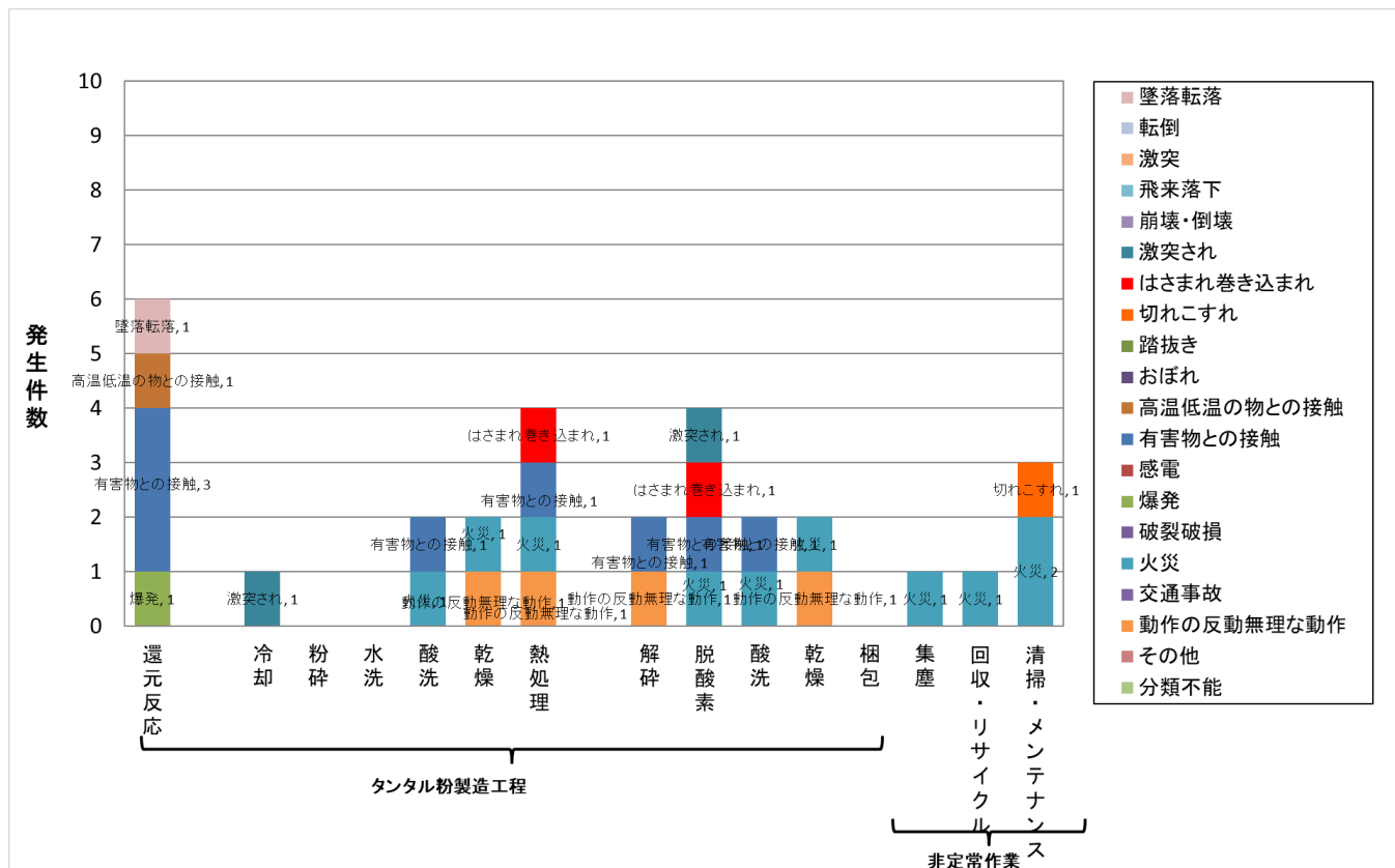
〔図Ⅱ-6-15 タンタル粉 工程別事故型リスク (2005 年～2022 年)〕
