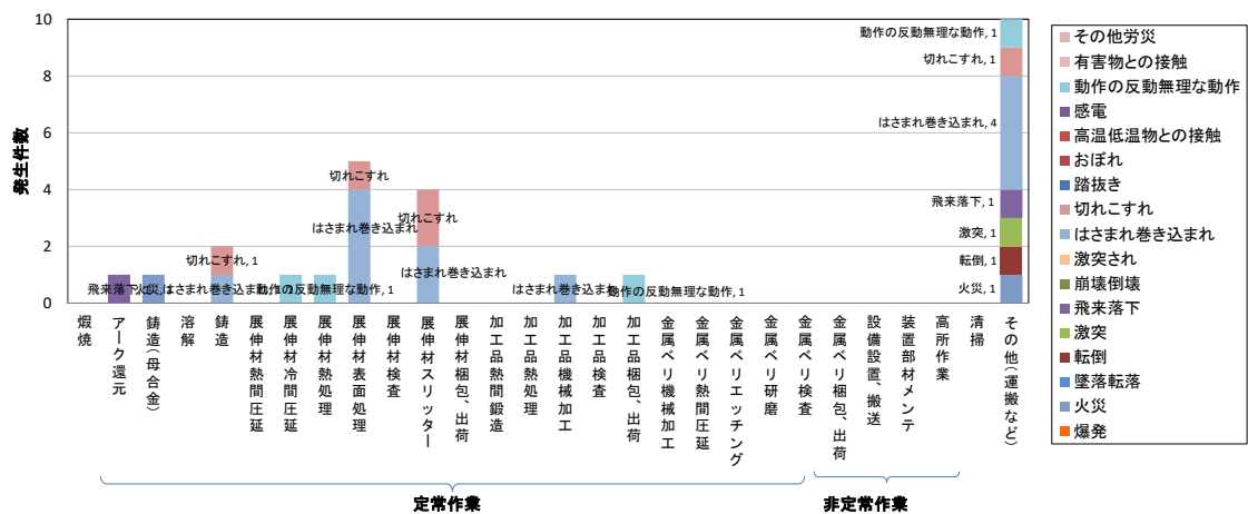
〔図Ⅱ-12-10 ベリリウム製造工程 工程別事故型発生件数(2005年～2022年)〕
