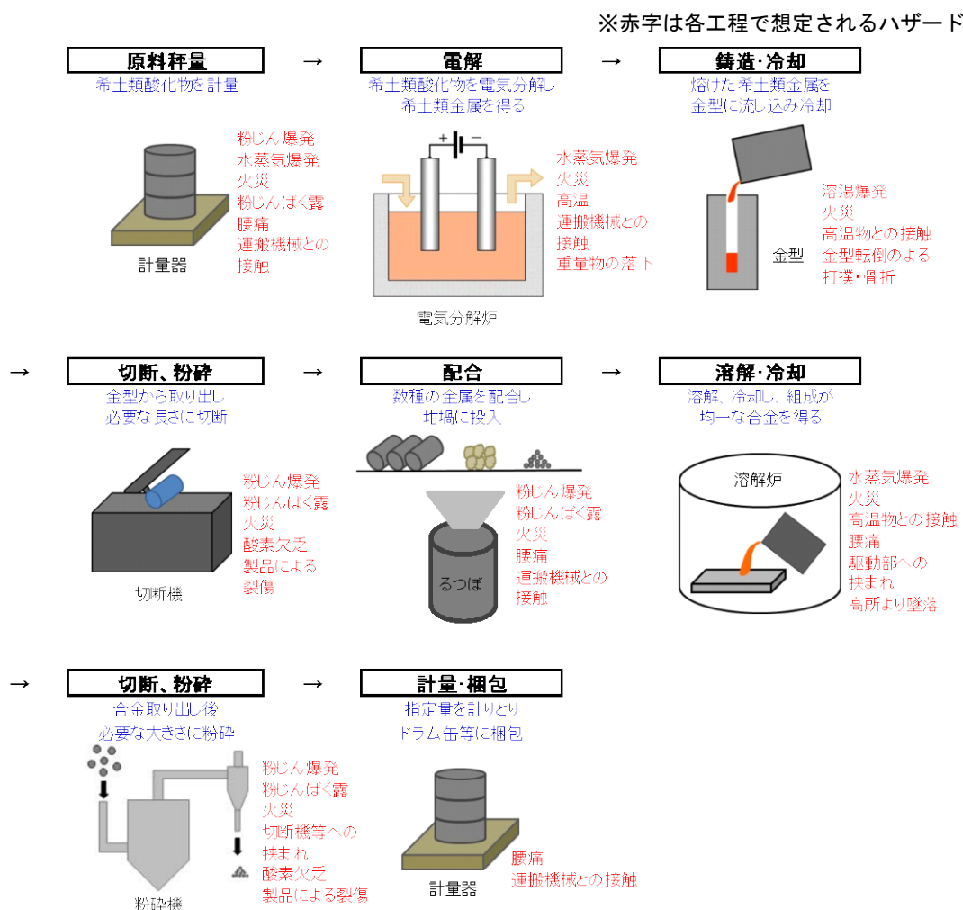
[図Ⅱ-4-13 金属・合金製造フロー]
