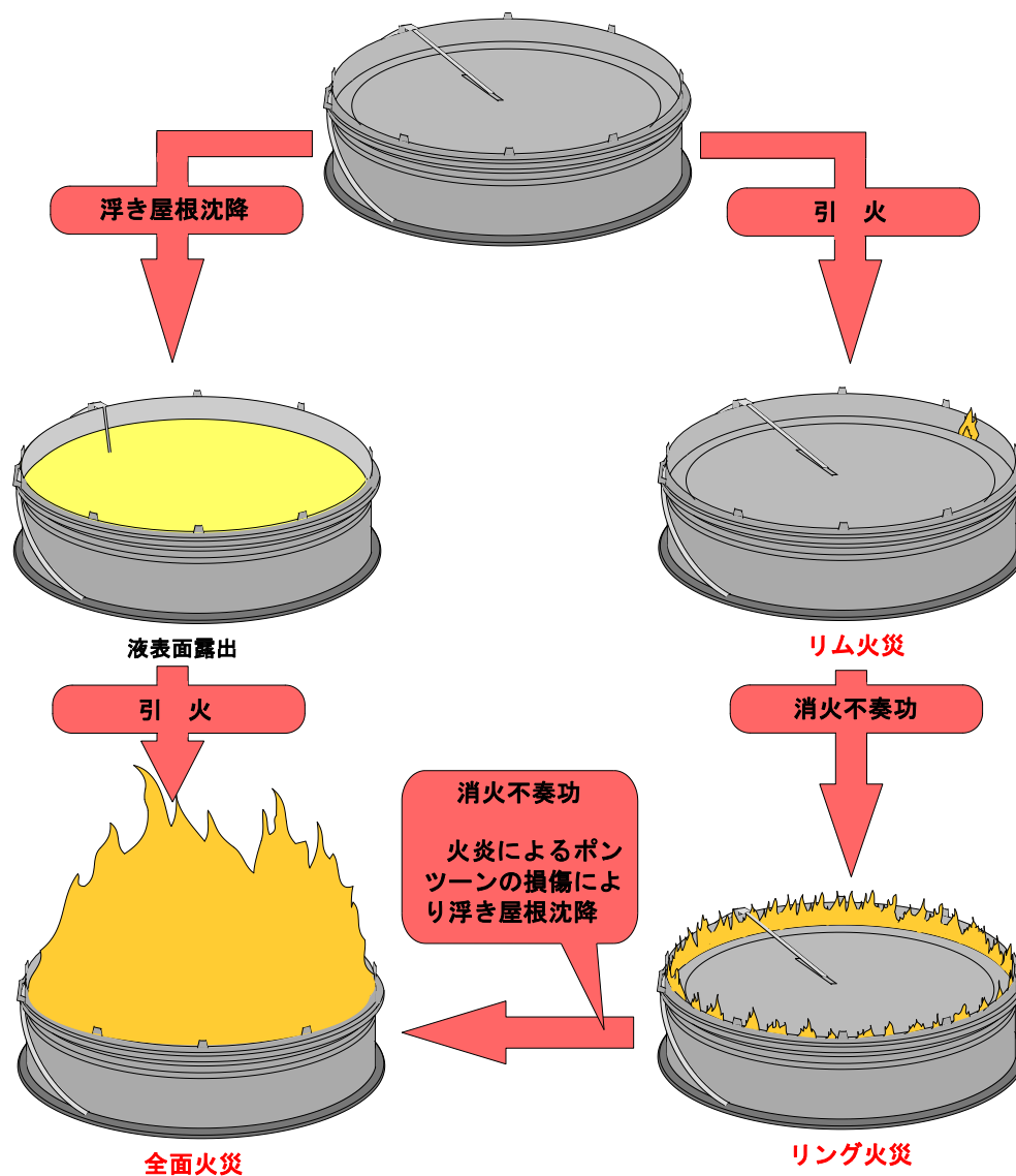
図2-2-2 浮き屋根式屋外貯蔵タンクの3つの火災形態の関連
