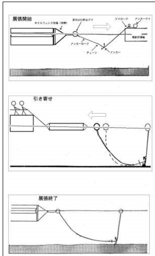
図 7-11-1 アンカリング方法
