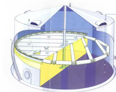
図 10-5-2 内部浮き屋根タンク構造図
