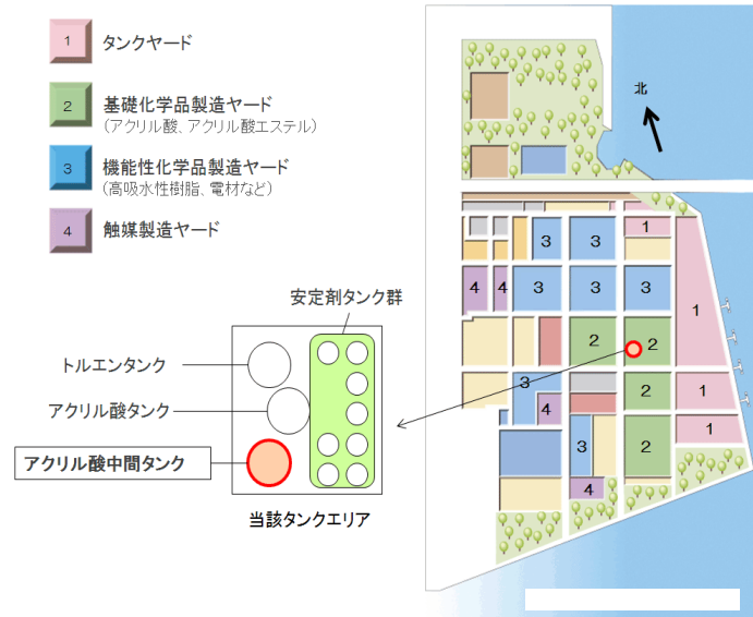
図 10-2-3 事業所配置図
