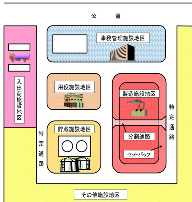
図5-1-1 施設配置図例
