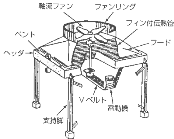
図5-2-5 エアファンクーラー
