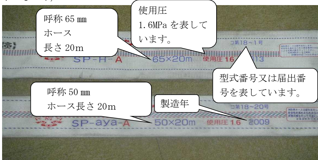
写真7-9-1 消防用ホースに表示された事項
