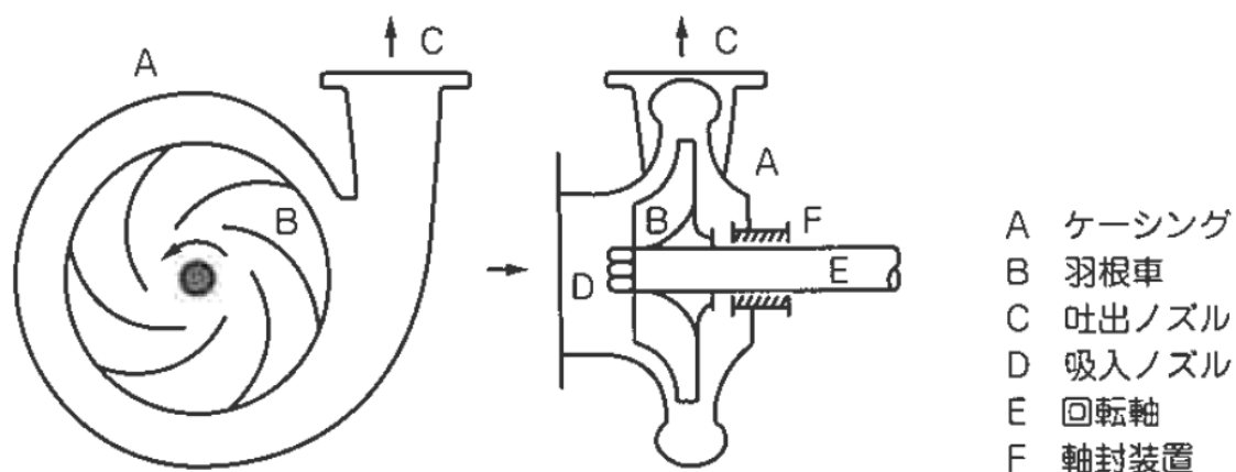
図5-2-2 遠心ポンプの構造
