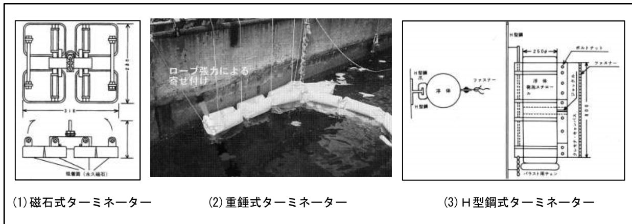
図 7-11-2 オイルフェンスの岸壁での係止方法
