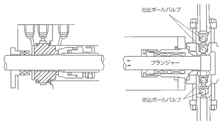
図5-2-3 メカニカルシールの構造（左）と 往復動ポンプ（右）
