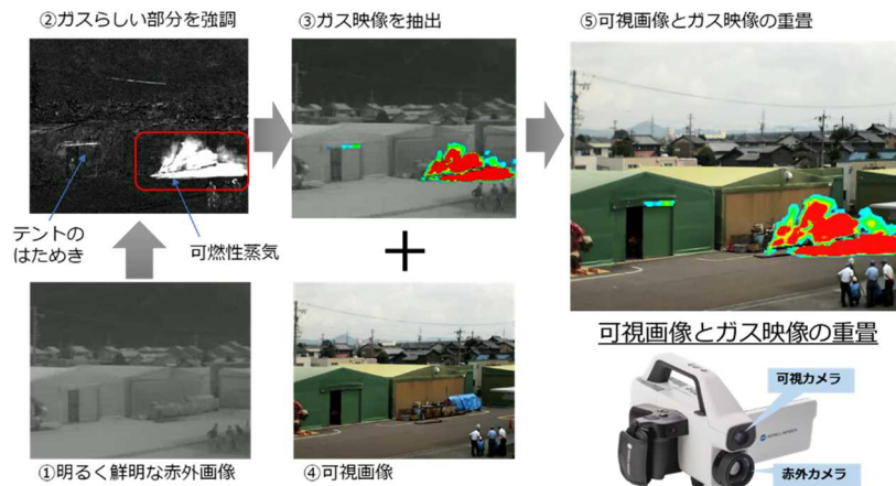
ガス監視カメラによる検知画面
