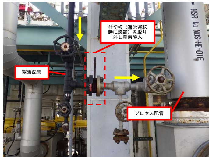
写真 8－3－14 窒素置換による引火防止措置
