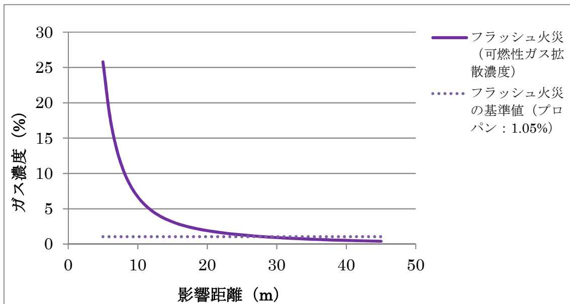
図2-3-1 プロパンの拡散火炎が伝ばし得る範囲の評価
