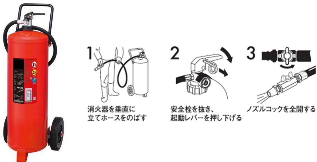
図 7－8－2 第 4 種の消火設備（粉末消火器の場合）
