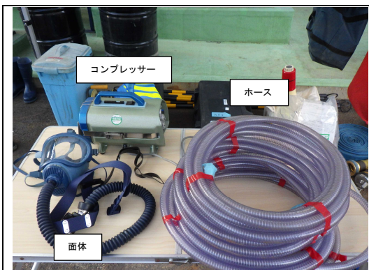
⑧エアラインマスク 危険性が高く、長時間の活動となる場合は、エアラインマスクを使用します。面体、ホース、コンプレッサーからなり、新鮮な空気を面体に送ります。
