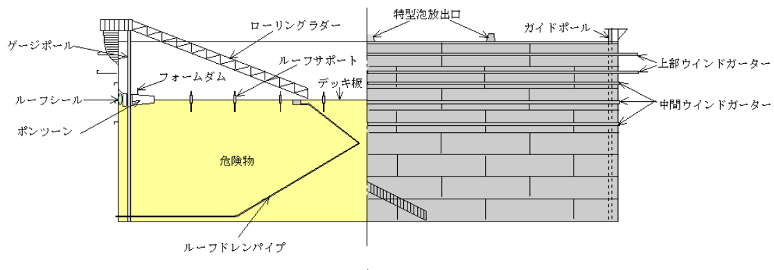
図2-2-3 浮き屋根式屋外貯蔵タンクの構造例
