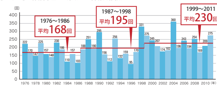
●1時間降水量50ミリ以上の年間観測回数は統計期間1976～2011年で増加傾向が明瞭に現れています。
