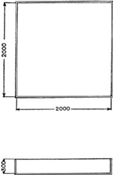
別図第3 B 火災模型（低発泡用）（第13条関係）
