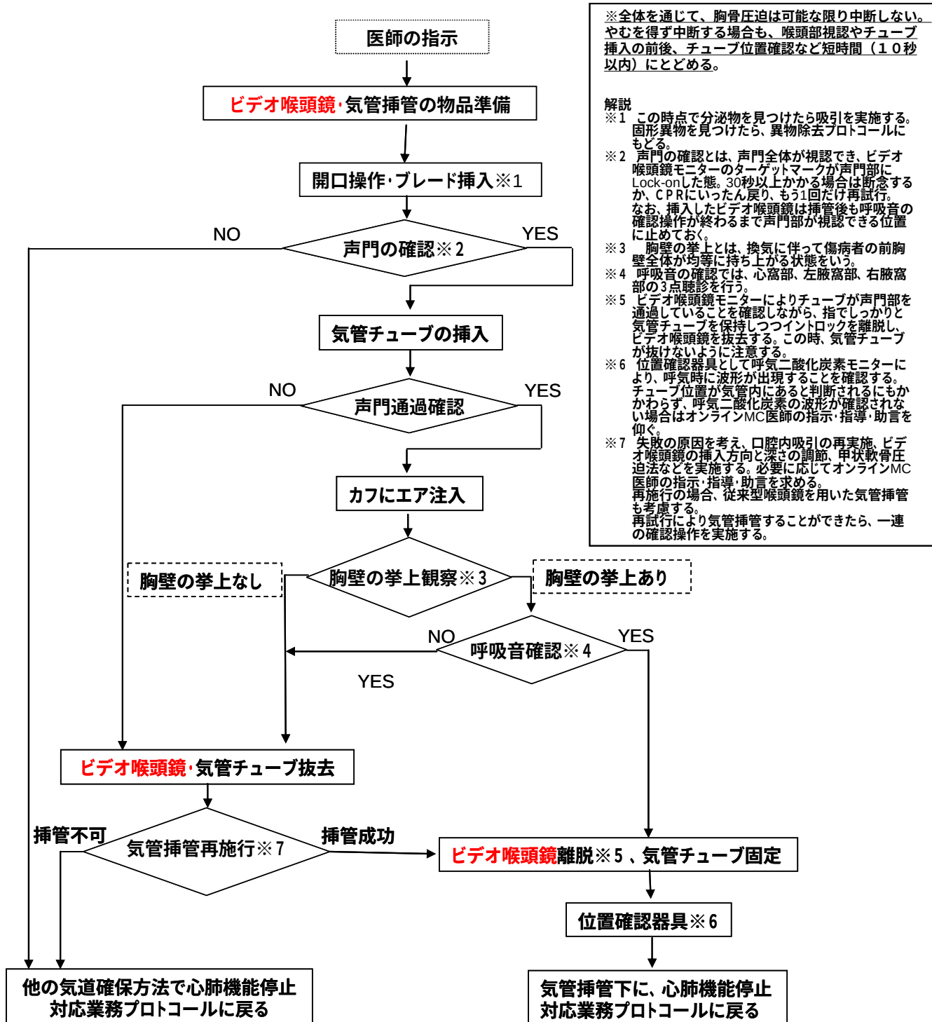
図 4-16 ビデオ喉頭鏡による気管挿管プロトコル（案）
