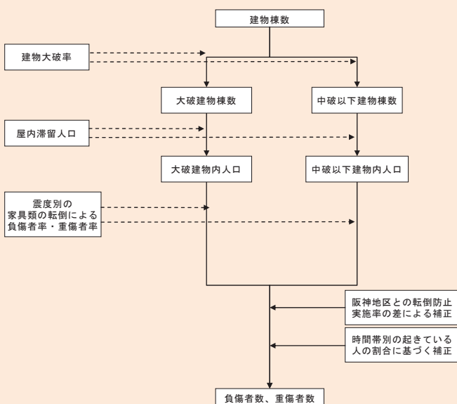
屋内転倒物による負傷者算定フロー
