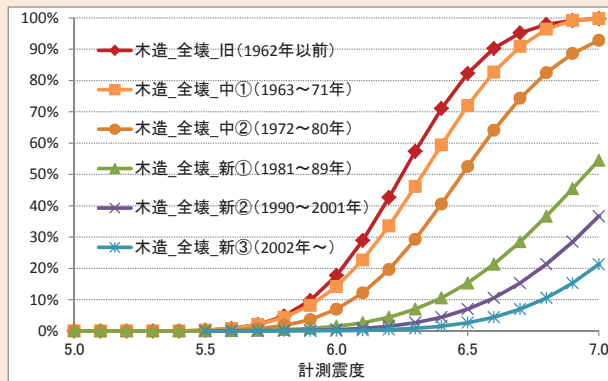
図 全壊率曲線(木造)
