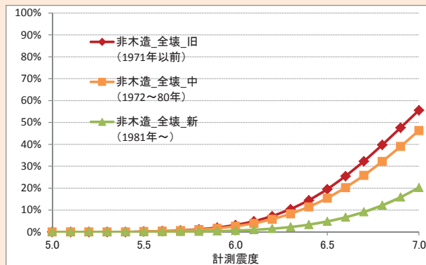
図 全壊率曲線(非木造)
