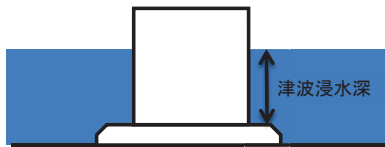
図 1 津波浸水深の定義
