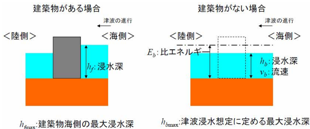
図 - 15 津波のせきあげ高を考慮した基準水位の設定
