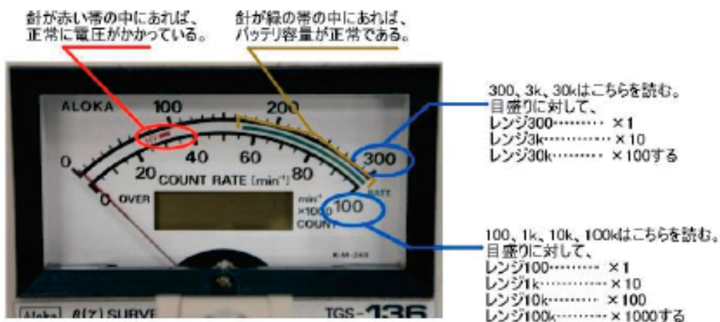
写真 2-4-1：GM 管式サーベイメータ
