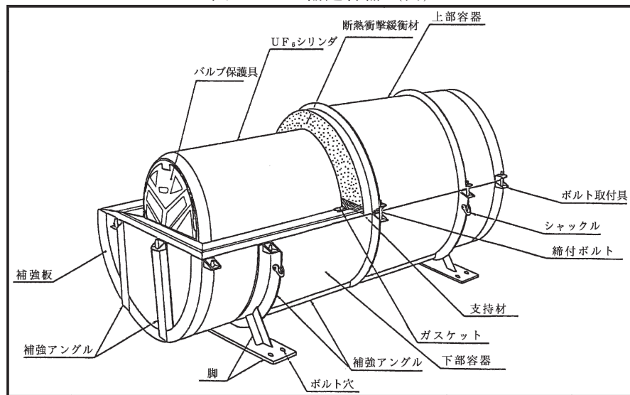
図 2-2-1：輸送容器（例）
