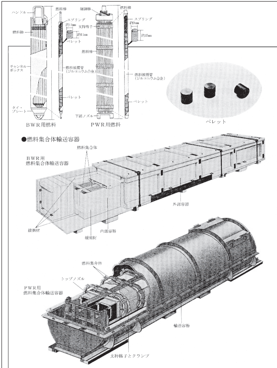
新燃料集合体の輸送容器（一例）
