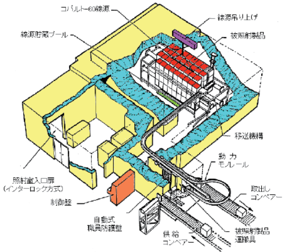
図 2-1-3: \gamma 線照射施設 (例)
