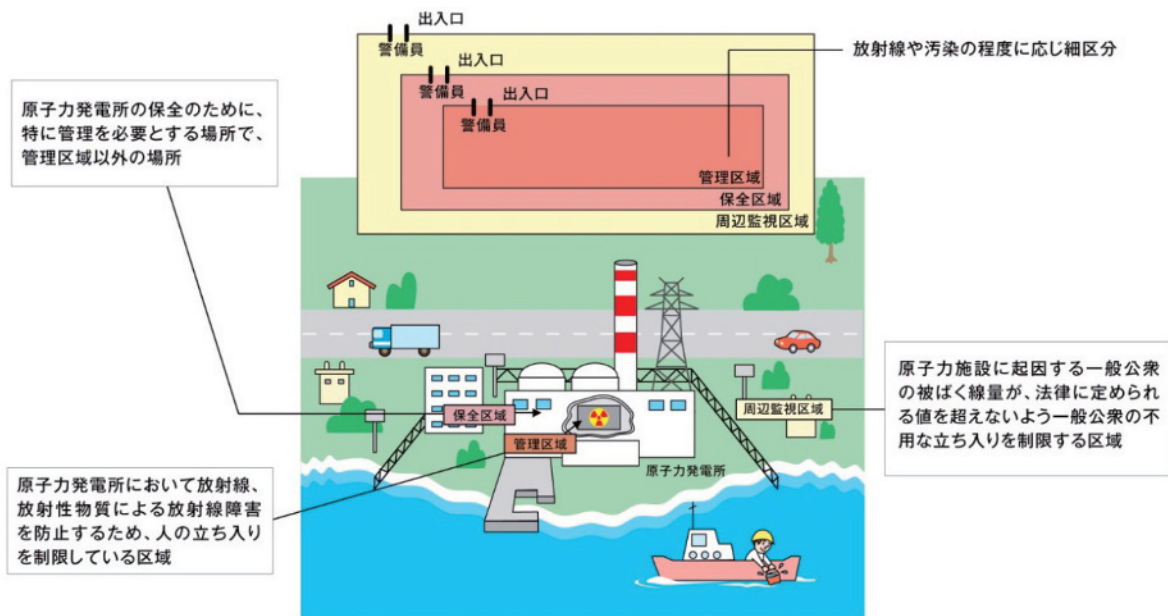
図 2-1-1：原子力発電所の区域区分
