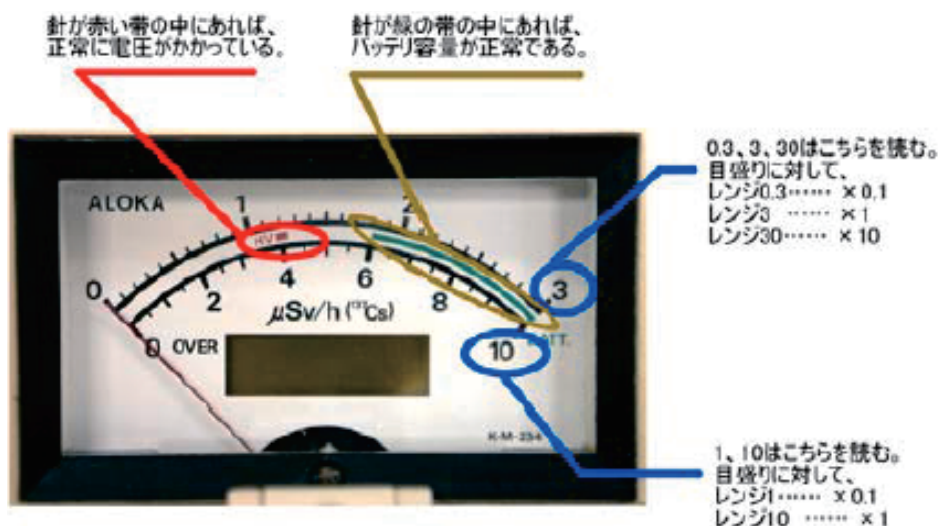
写真 2-4-2：【参考】 NaI シンチレーション式サーベイメータ（空間線量計）
