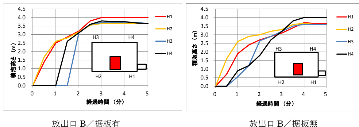
図 3-15 積泡高さの計測値
