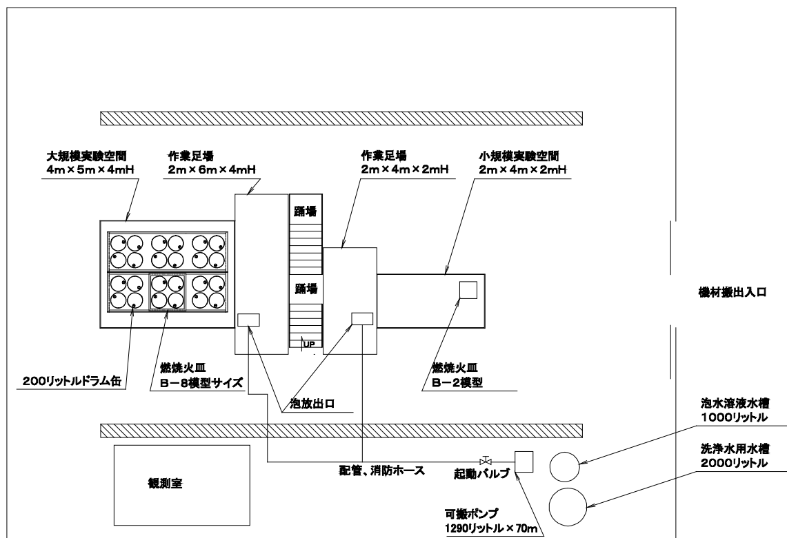
実験施設全体配置図（平面図）
