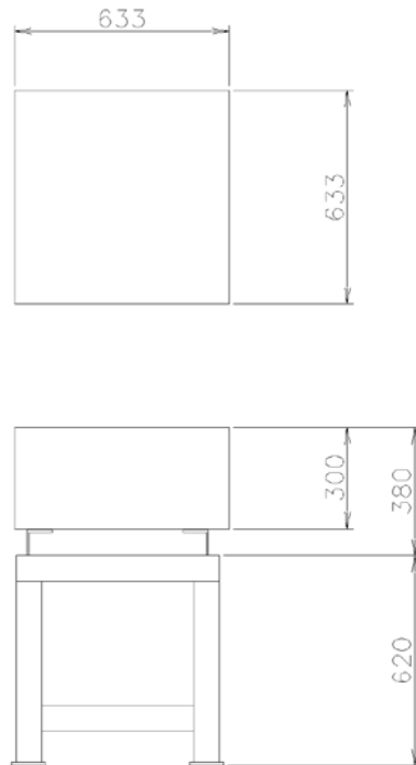
図 3－4 火災模型
