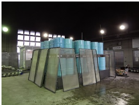
ラック及びドラム缶（組立中）
