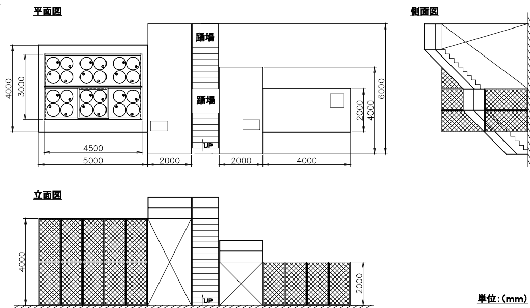
実験施設主要寸法図（3面図）
