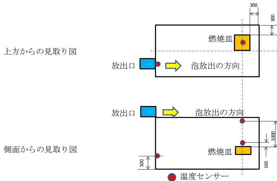
図 3 - 5 温度計測位置
