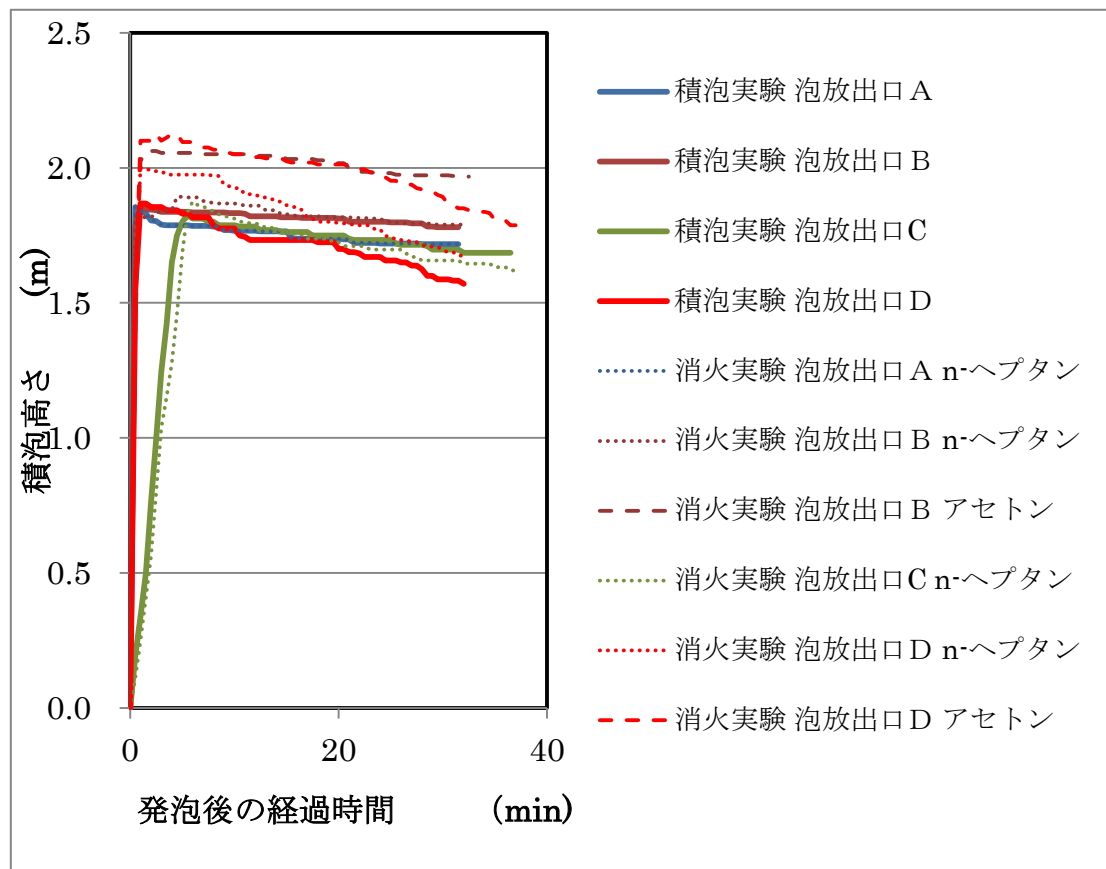
図 3-10 発泡後の積泡高さの変化
