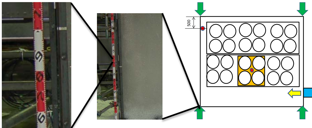
図 3-14 積泡高さの計測位置
