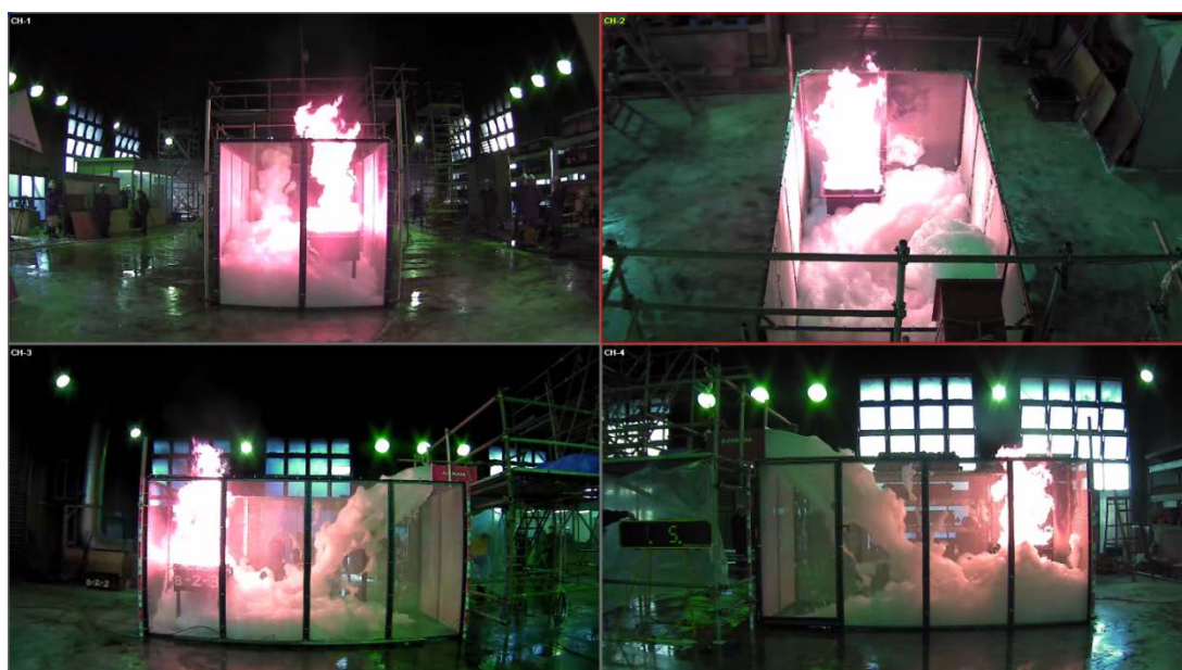
監視カメラ画像の例 (21-3 小規模区画 B 泡放出口 n-ヘプタン 泡放射 5 秒後) 画像ファイル h264 形式、1920*1080、7 コマ/秒
