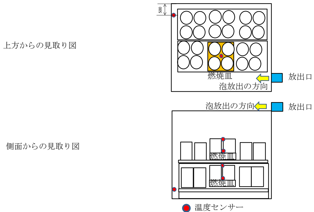
図 3－13 温度センサー配置図
