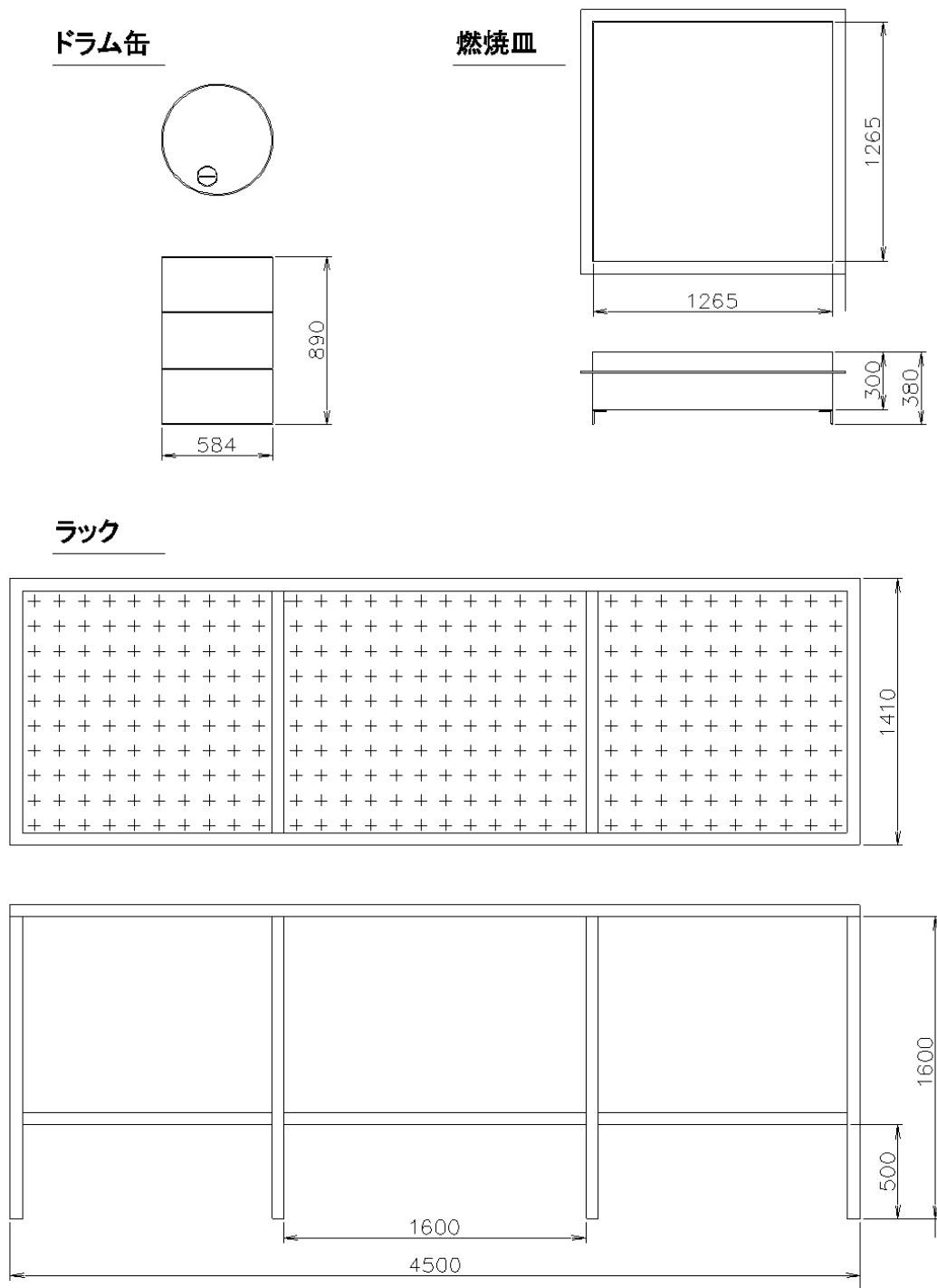
図 3 - 1 1 ドラム缶、燃焼皿、ラックの寸法
