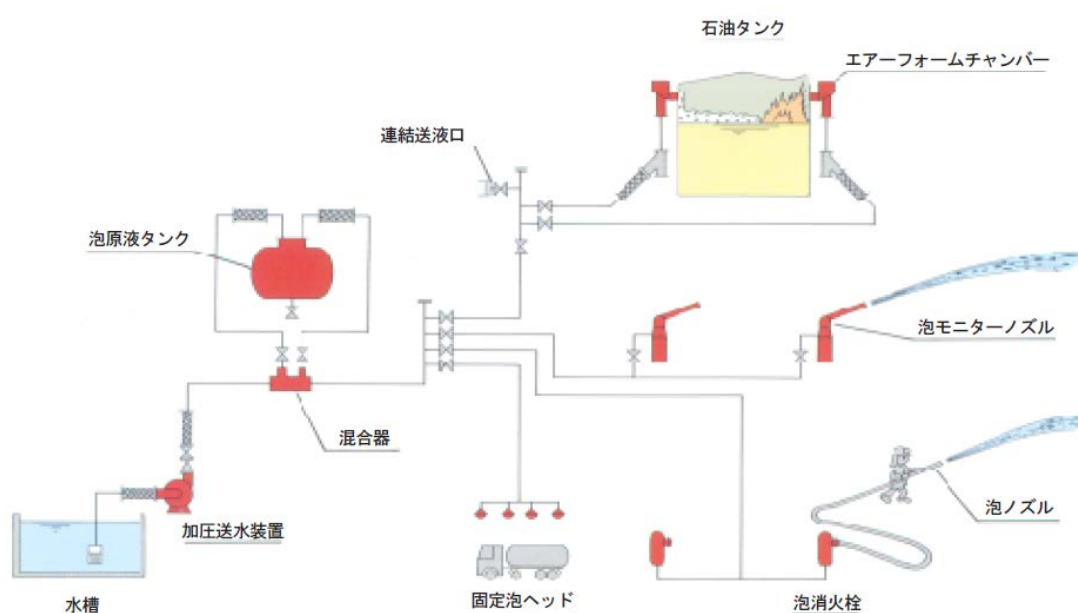
図2-1 泡消火設備の構成（深田工業(株)ホームページより）
