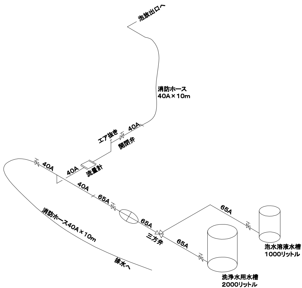
配管構成の概要図
