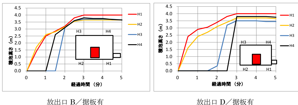
図 3-16 積泡高さの計測値
