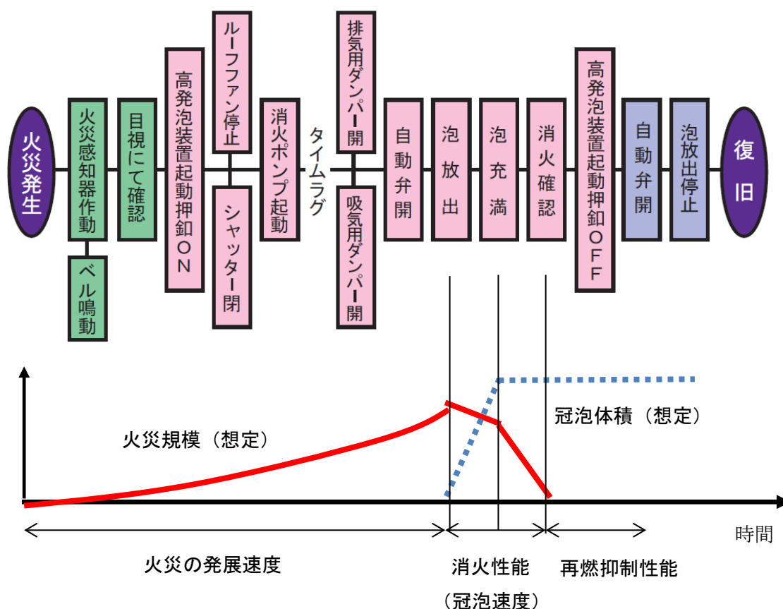
図3-1 非常時の操作と火災の発展速度の想定
