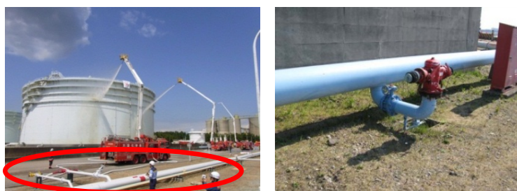
図2-1 消火用屋外給水施設の例（消火栓・配管）（○の部分）
