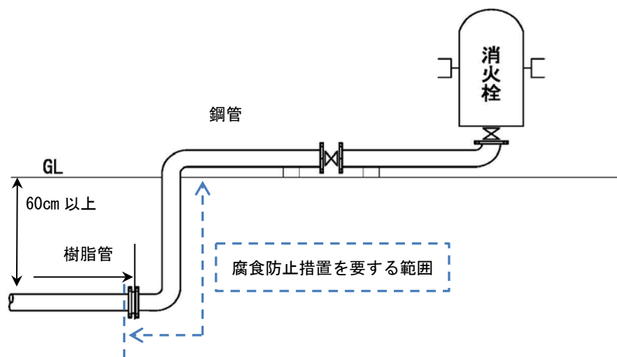
図4-7 施工例イメージ3
