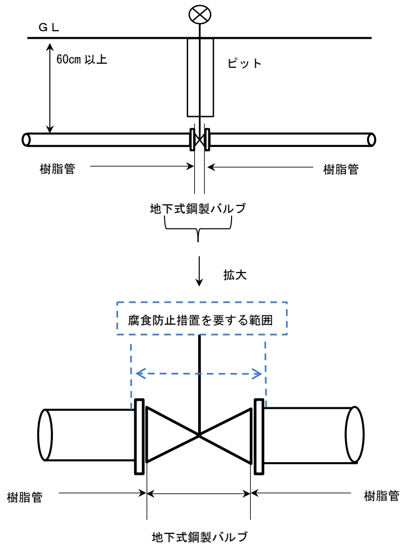
図 4 - 1 0 施工例イメージ 6
