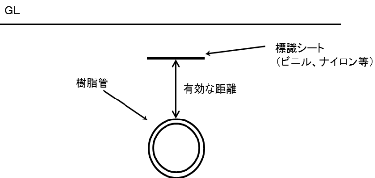
図 4 - 4 埋設位置標識 (地中) 埋設例
