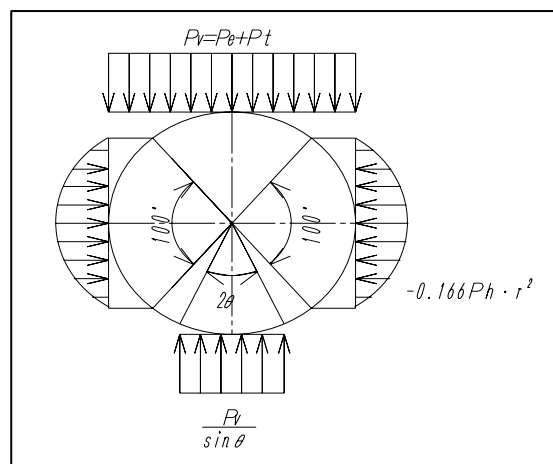
図-2 スパングレーの土圧分布図
