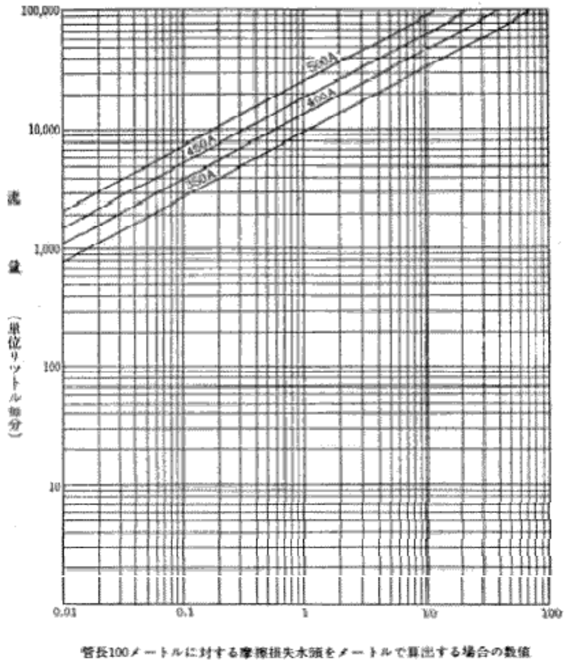
別図第4 配管用アーク溶接炭素鋼鋼管（日本工業規格G 3 4 5 7）の呼び 厚さ9.5ミリメートルである場合
