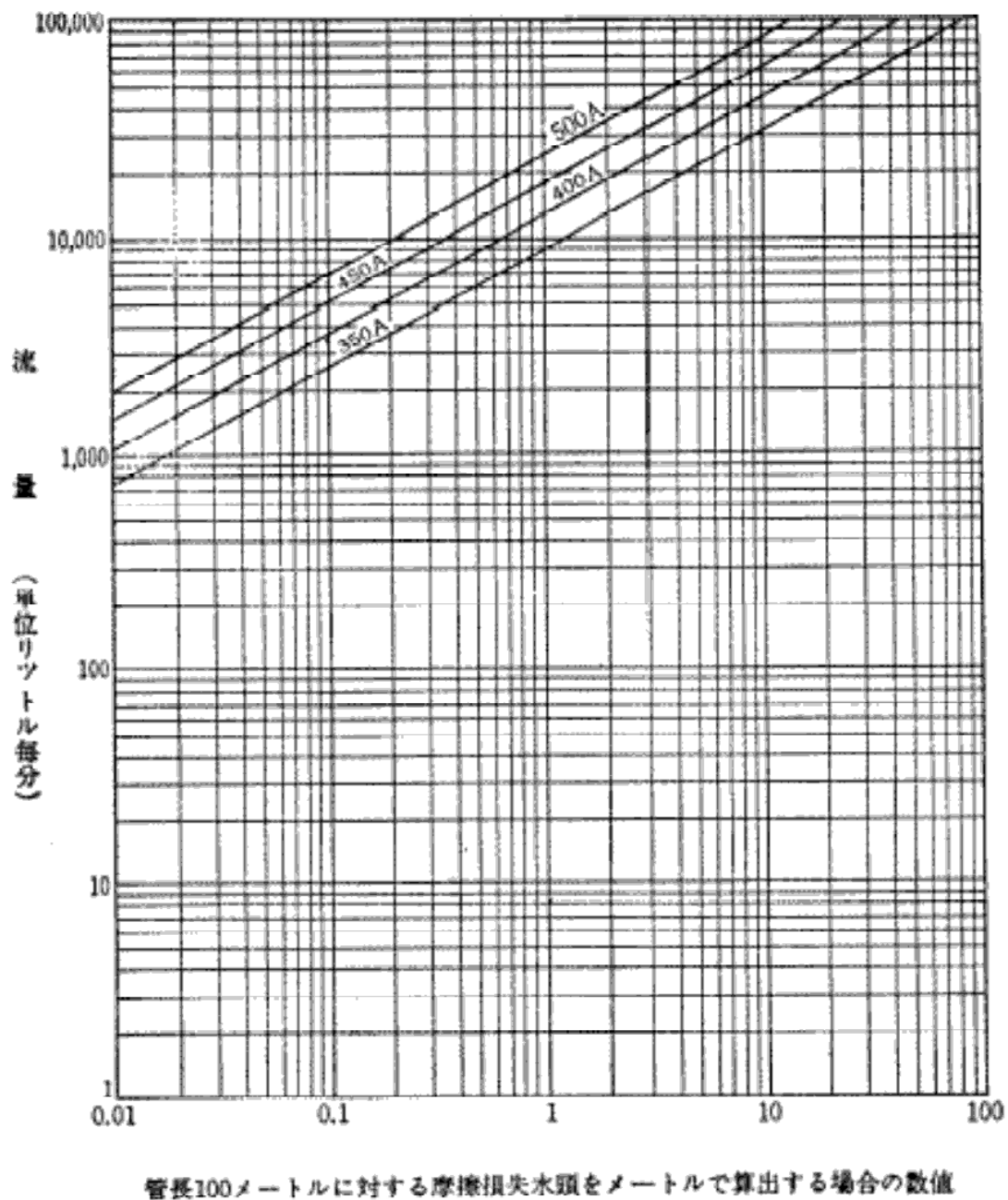
別図第5 配管用アーク溶接炭素鋼鋼管（日本工業規格G 3 4 5 7）の呼び 厚さ12.7ミリメートルである場合
