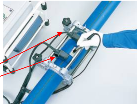
同種管の E F 接合例 (例)
