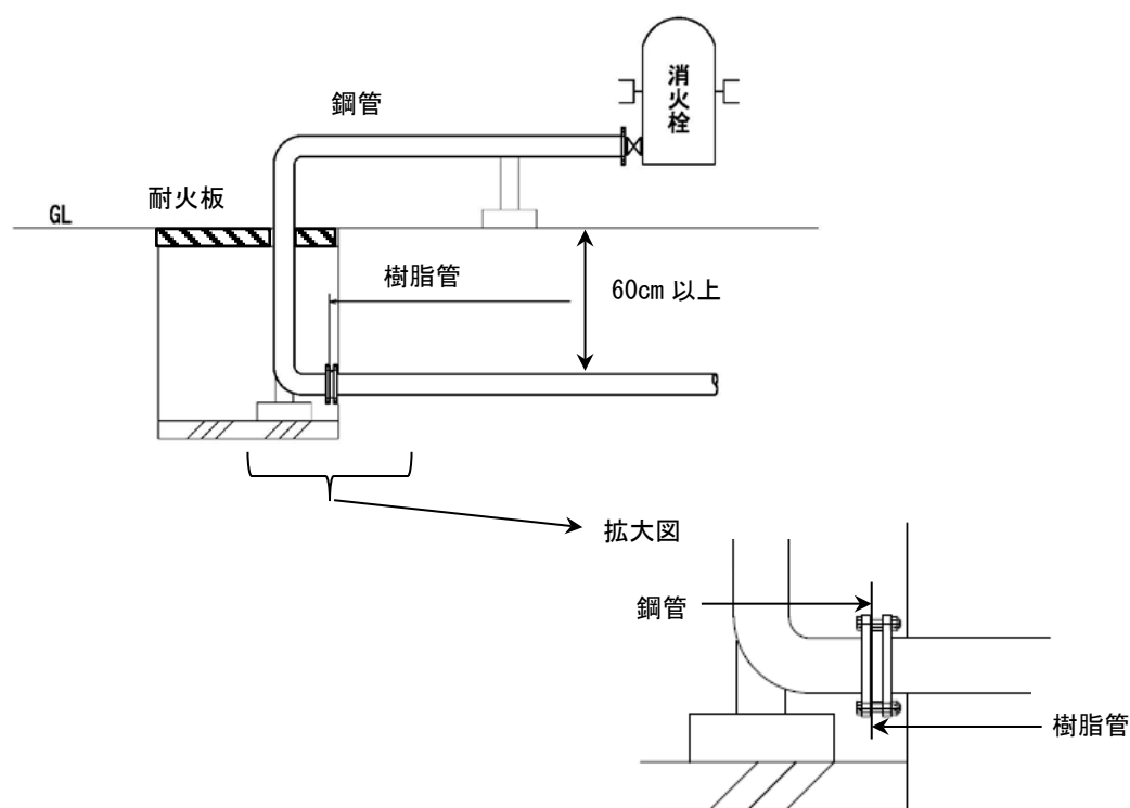
図4-5 施工例イメージ1
