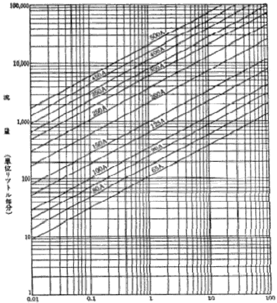
別図第3 圧力配管用炭素鋼鋼管（日本工業規格G 3 4 5 4）スケジュール 80である場合
