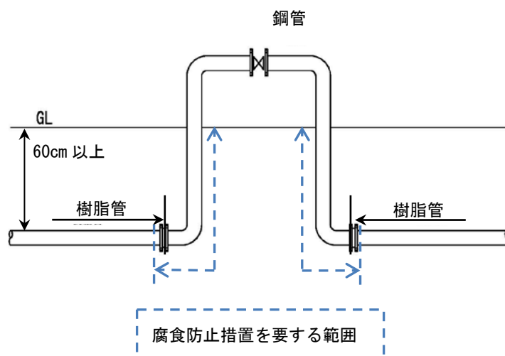
図 4-9 施工例イメージ 5
