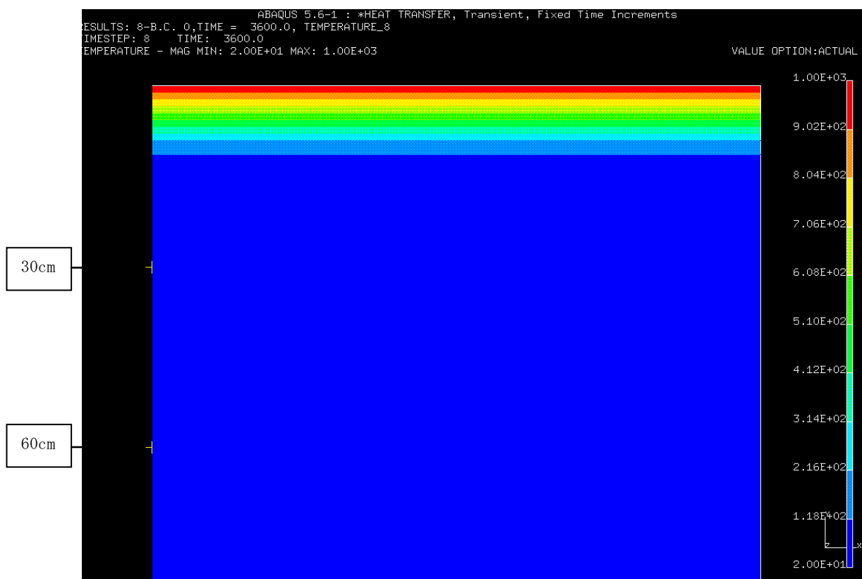
図－３ FEM解析結果（１時間後の温度分布）
