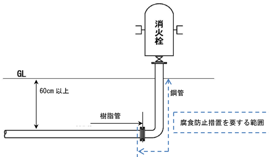
図 4-8 施工例イメージ 4
