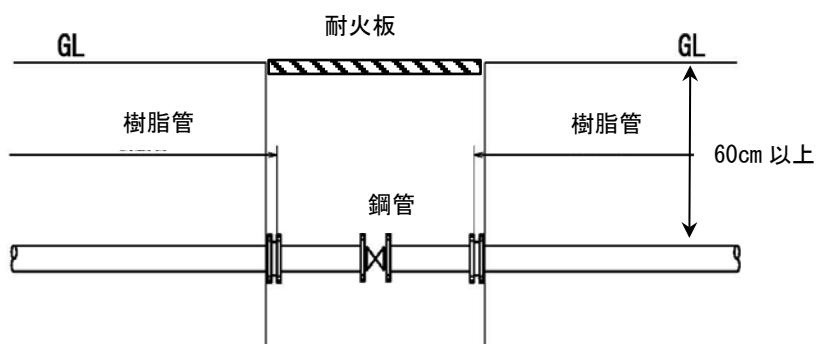
図4-6 施工例イメージ2
