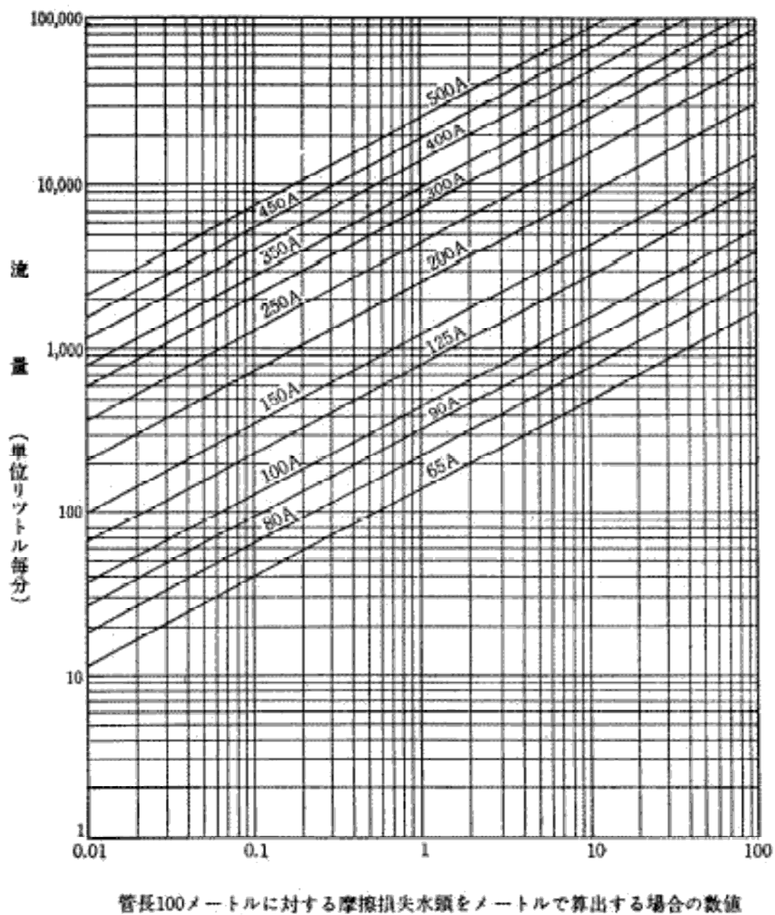
別図第1 配管用炭素鋼鋼管（日本工業規格G 3 4 5 2）及び配管用アーク 溶接炭素鋼鋼管（日本工業規格G 3 4 5 7）の呼び厚さ7.9ミリメートルである場合
