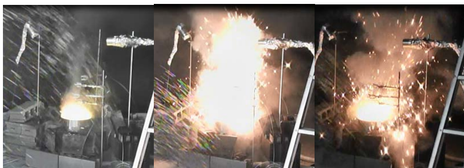
ペール缶内で燃焼中のマグネシウム等の切削屑に直状放水を行った様子
