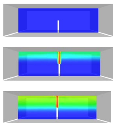
水素ガス濃度分布シミュレーション
