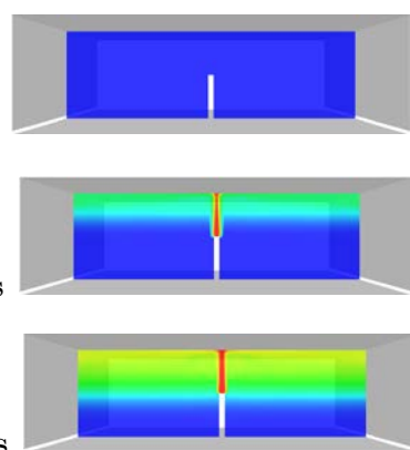
アンモニアガス濃度分布シミュレーション
