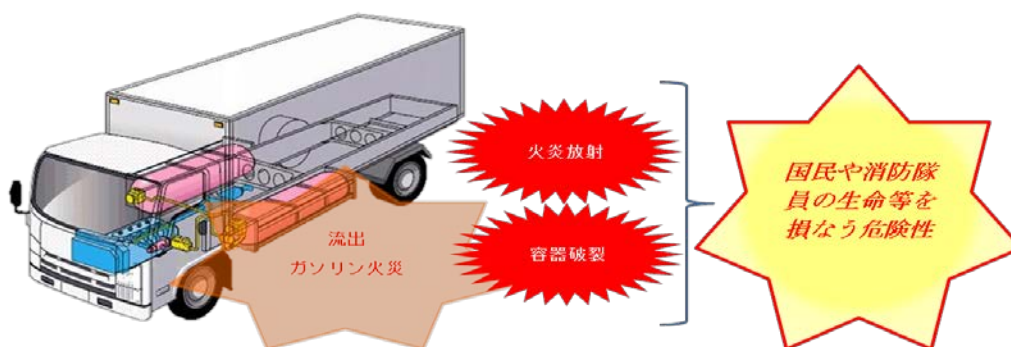
図9 天然ガス自動車の下部にガソリンが流れ込んで火災となる場合の危険性
