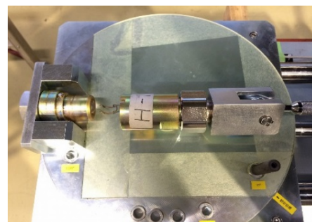
図 22 緊急離脱カプラー離脱試験
