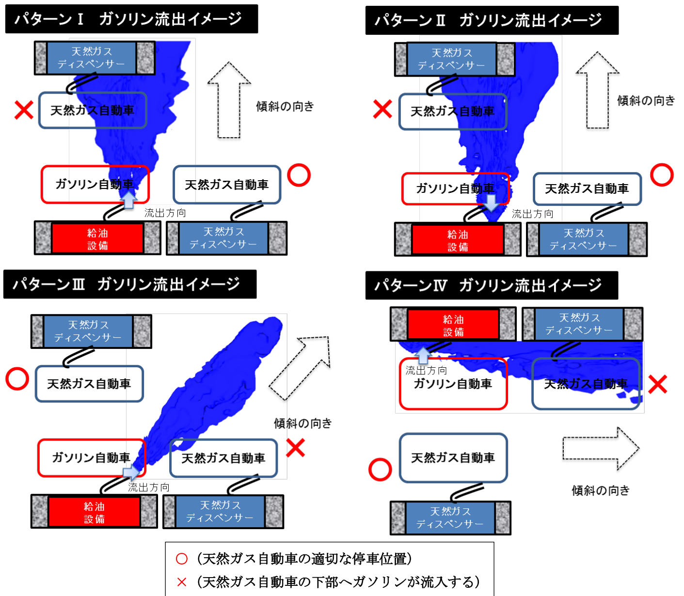
図 34 各パターンのガソリン流出イメージ
