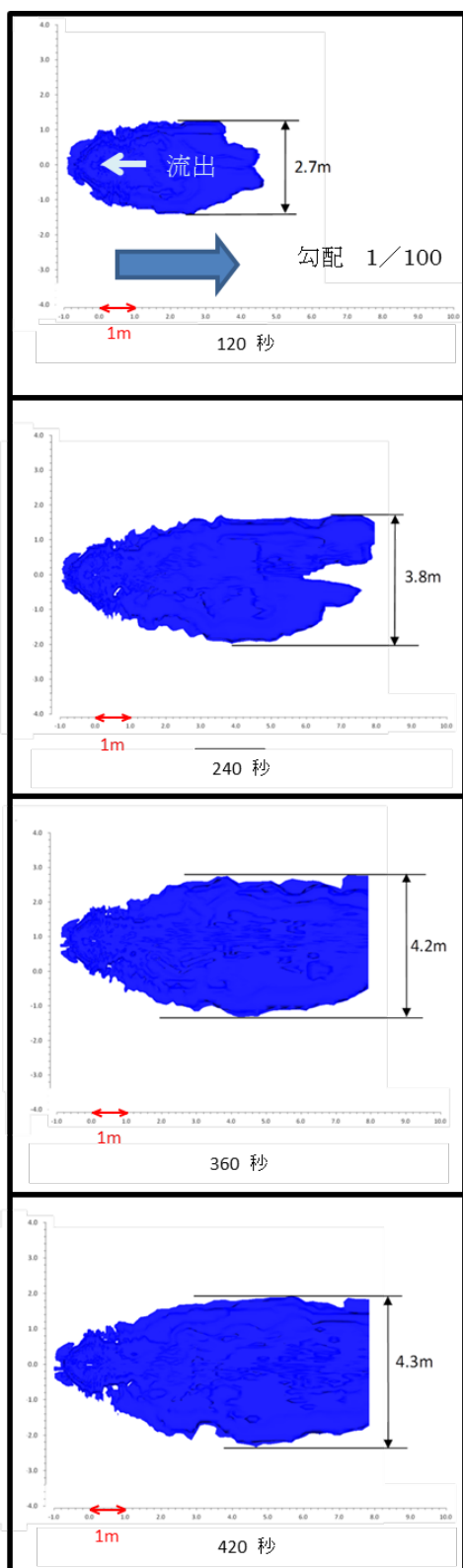
図 28 パターンⅡ－1 計算結果
