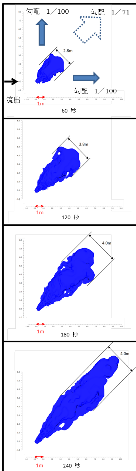
図 30 パターンⅢ－１計算結果
