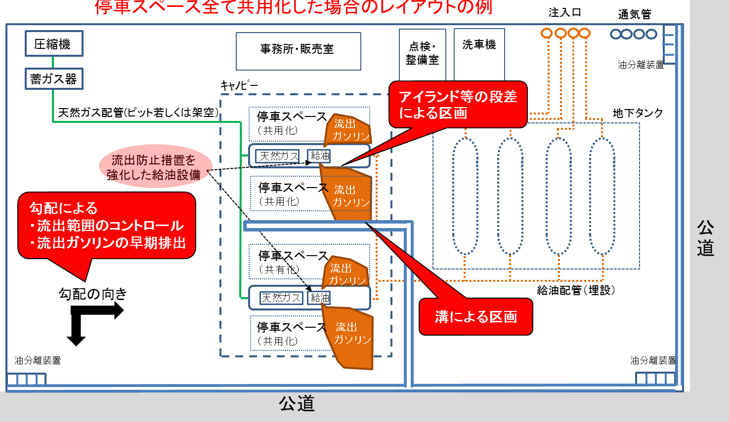
図 42 想定されるレイアウト 傾斜と溝を設ける場合
