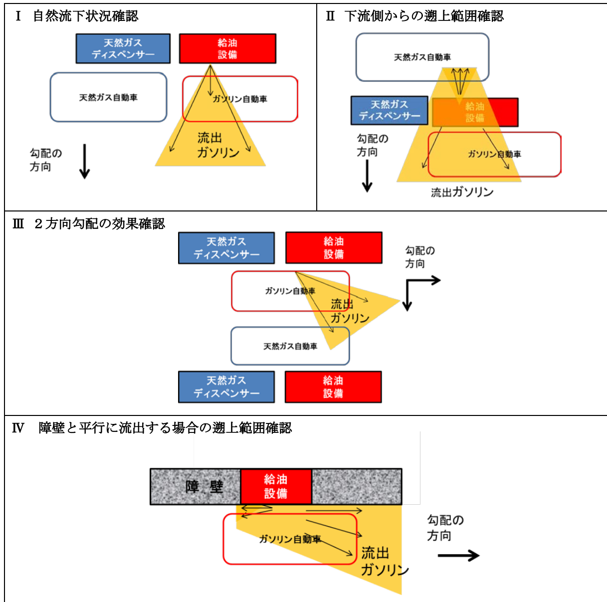
図 24 想定する流出イメージ図
