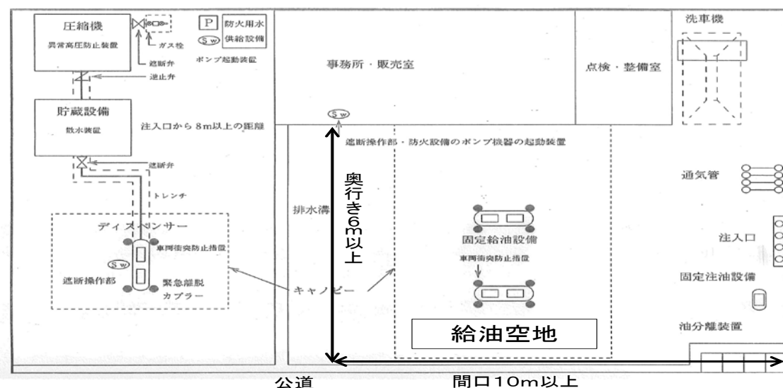
図2 天然ガスタンド併設給油取扱所のモデル図
