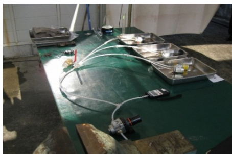
図 20 使用した試験装置
