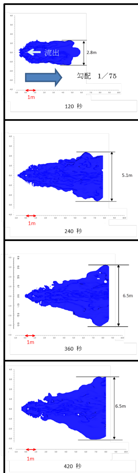
図 29 パターンⅡ－2 計算結果
