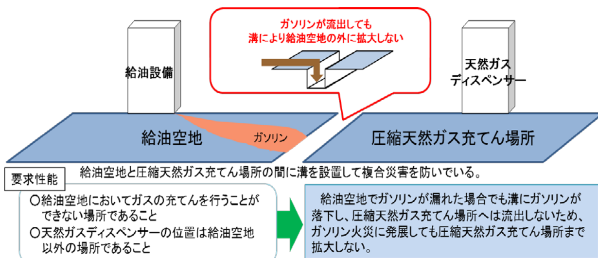
図8 消防法令における天然ガスタンク併設給油取扱所の防火安全対策（現状）
