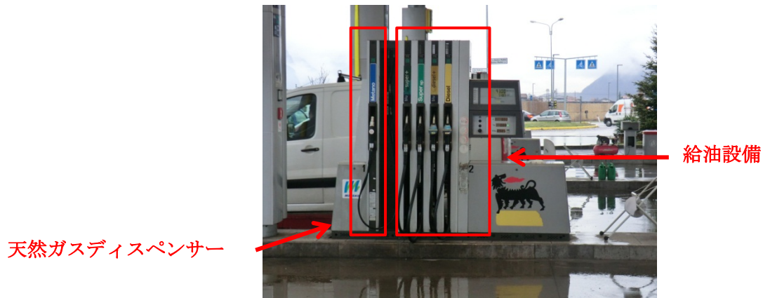
図5 給油設備と天然ガスディスペンサーが一体となったマルチディスペンサー（MD）の設置例（イタリア）
