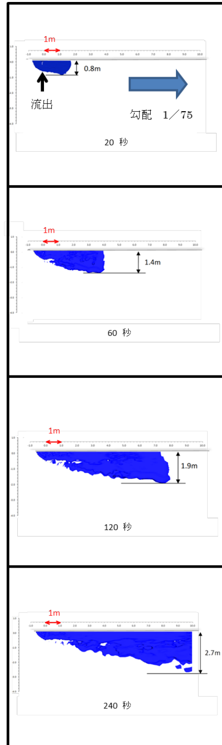
図 33 パターンⅣ－２ 計算結果
