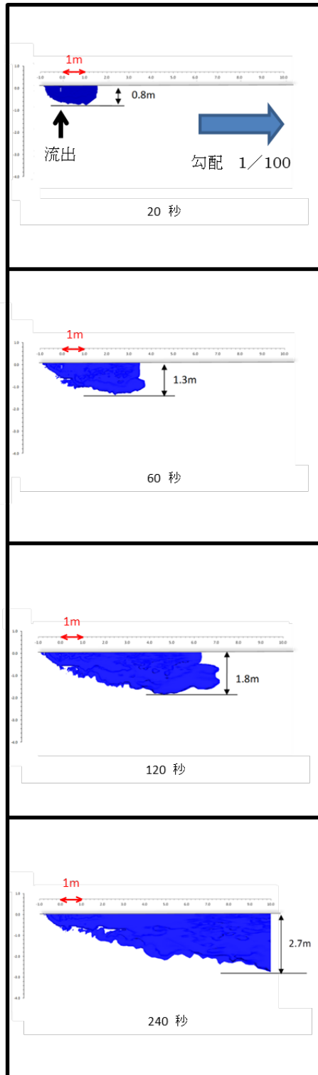
図 32 パターンⅣ－１ 計算結果
