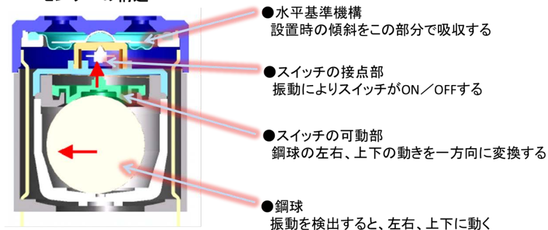
図 36 感震装置の構造例（提供：日本ガソリン計量機工業会）
