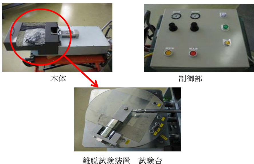
図 19 使用した試験装置
