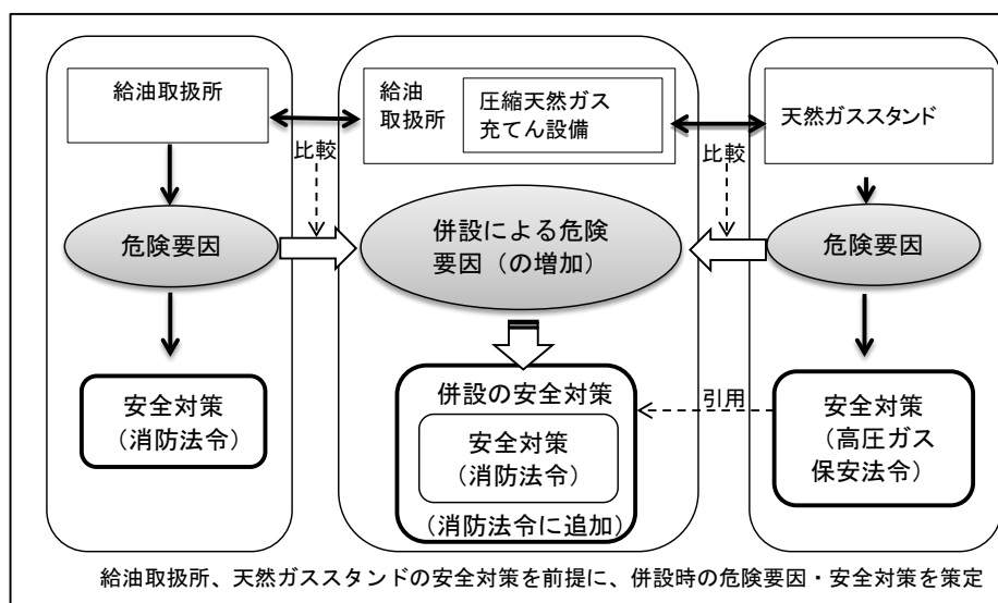
図3 天然ガス設備設置給油取扱所の安全対策の考え方（概念図）
