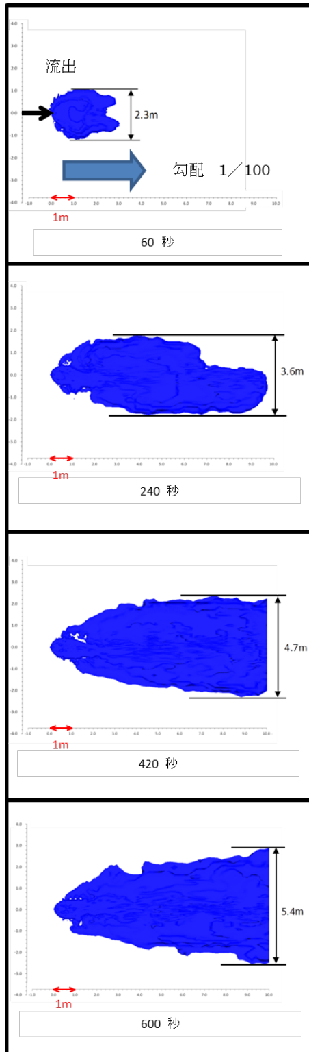
図 26 パターン I-1 計算結果
