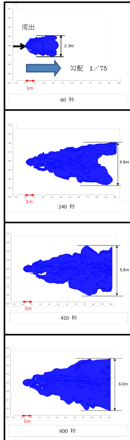
図 27 パターン I-2 計算結果
