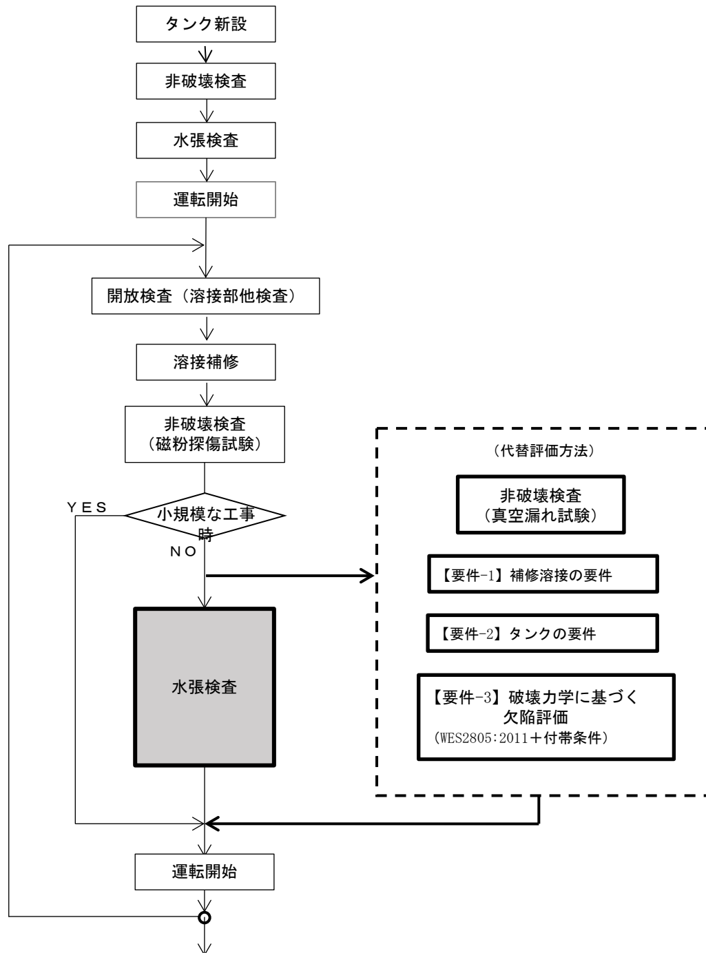
図 水張検査の代替評価イメージ
