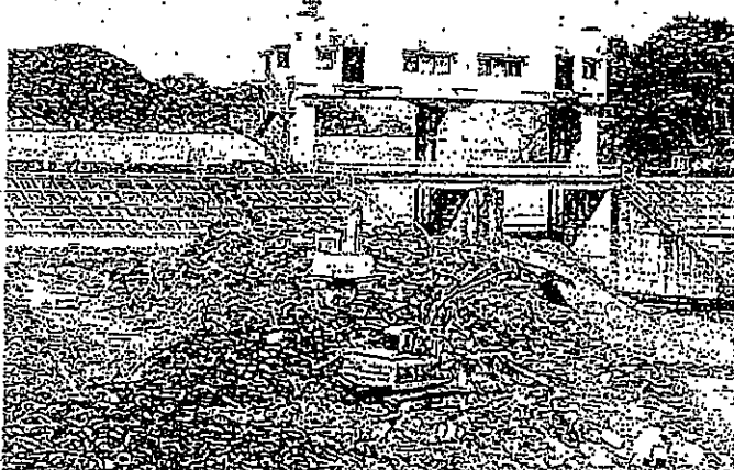
遠隔操作できずに消防団員が現場で手動閉鎖した水海水門—岩手県釜石市両石町で
