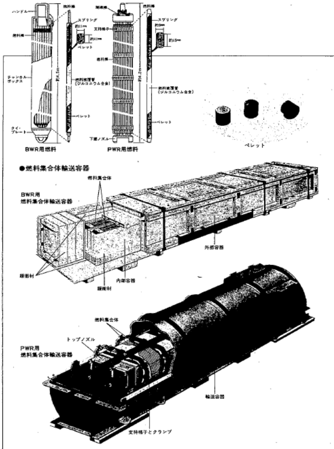
新燃料集合体の輸送容器（一例）
