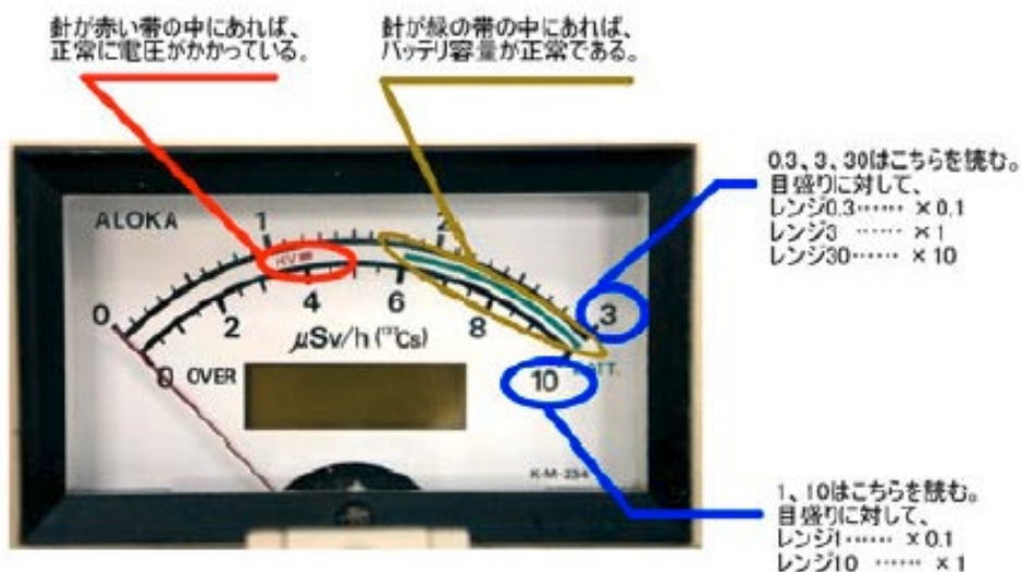
写真 2-4-2：【参考】NaI(Tl)シンチレーション式サーベイメータ（空間線量計）
