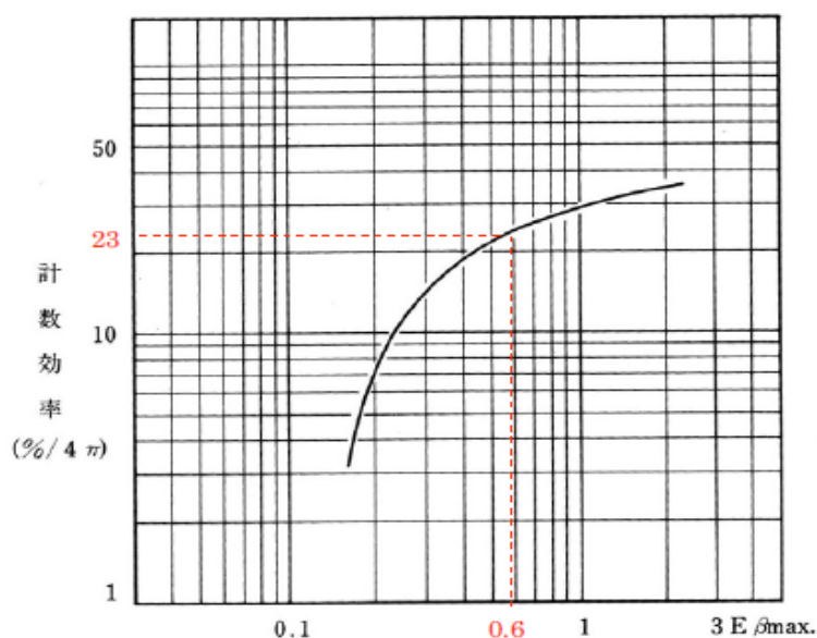
\beta 線最大エネルギーに対する計数効率 (TGS-133 型)
