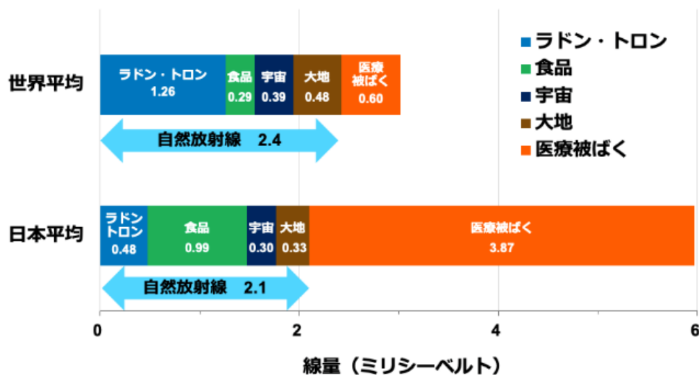
図 1-2-2：日常生活における被ばく（年間）
