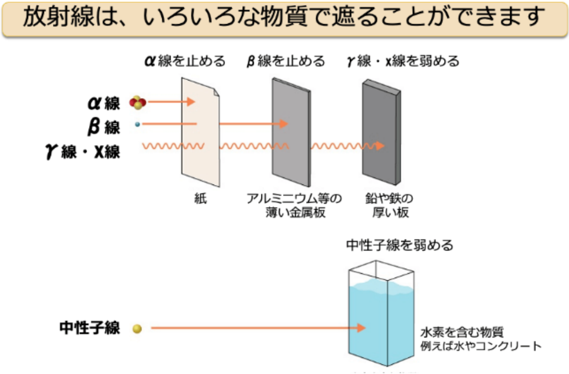
図 1-1-1：主な放射線の透過力と被ばくの特徴
