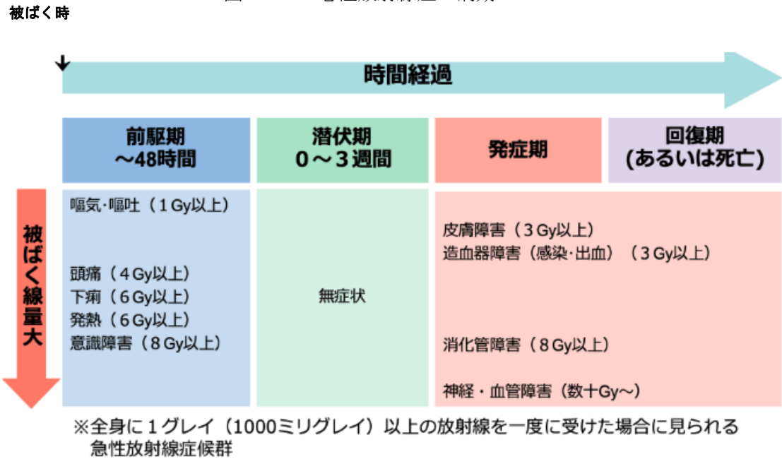
図 1-2-3：急性放射線症の病期
