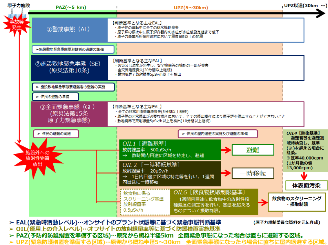
図4-1 発電用原子炉に係る緊急事態の区分とEAL・OILに基づく防護措置
