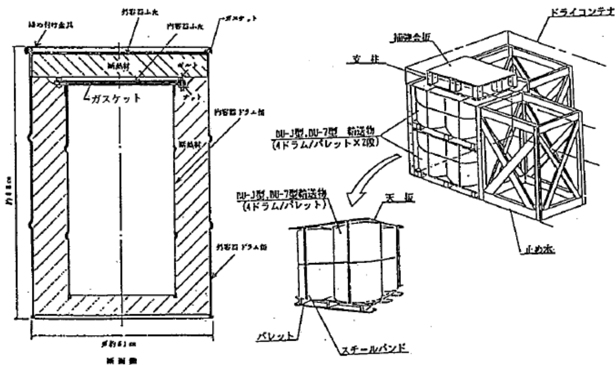
固縛の一例
