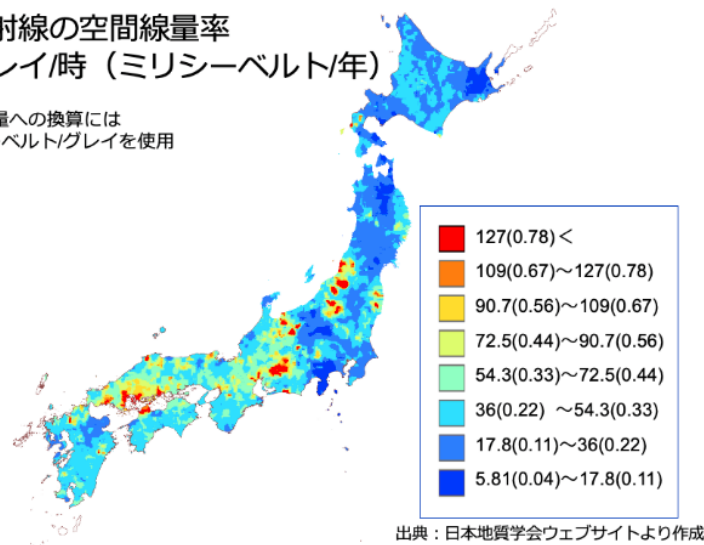
図 1-1-4：自然放射線の空間放射線量率 ナノグレイ/時（ミリシーベルト/年）
