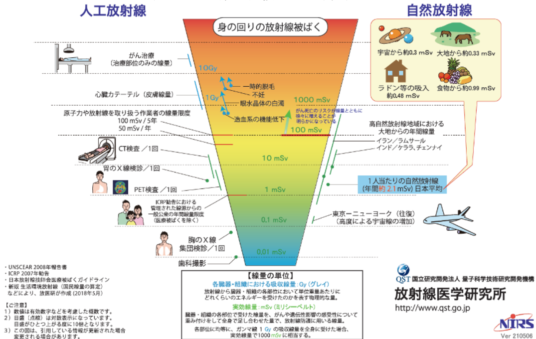
図 1-1-3：放射性被ばくの早見図
